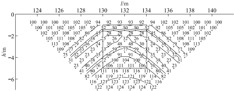
图 3 模型 2 偶极—偶极视电阻率等值线(单位:Ω·m) Fig. 3 Dipole-dipole apparent resistivity contour of model 2
