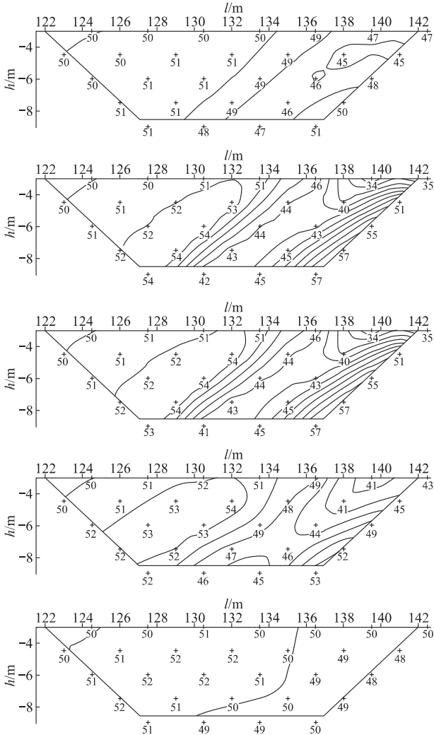
图 5 模型 3 沿 y 方向断面视电阻率等值线(单位:Ω·m) Fig. 5 Apparent resistivity contour of model 3 in the y direction
