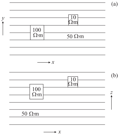
图 4 模型 3 的平面及剖面示意 Fig. 4 Plane and sectional sketch map of model 3 a. 平面示意图;b. 剖面示意图
