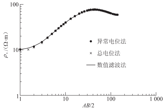
图 2 有限元法与数值滤波法结果对比
