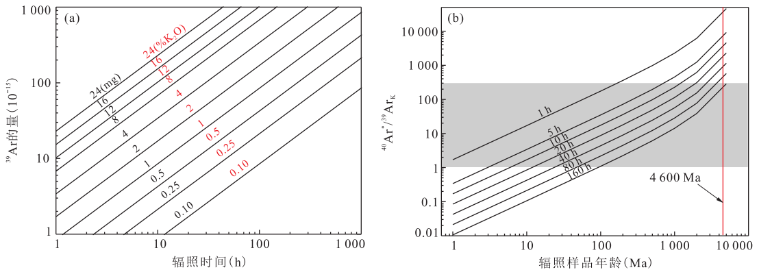
图 3 39 Ar K 产率曲线(a)和不同年龄样品的辐照时间与 40 Ar* / 39 Ar K 值关系(b)
