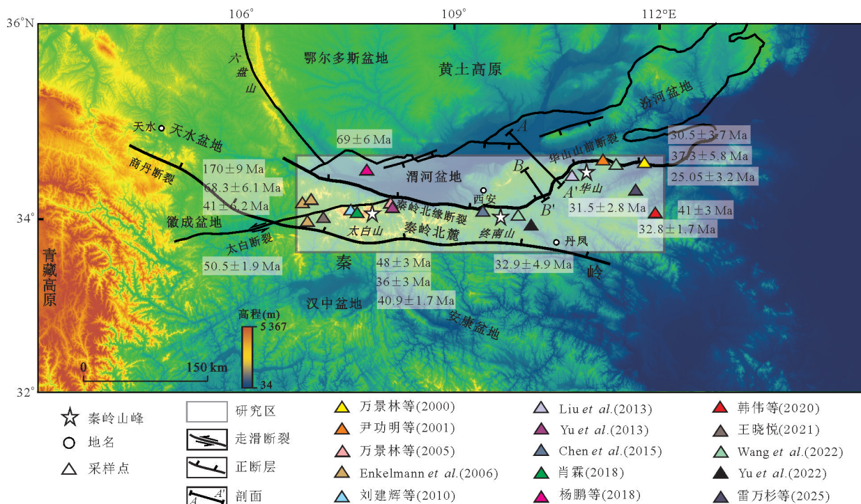
图 1 秦岭北麓及周边地区数字高程
