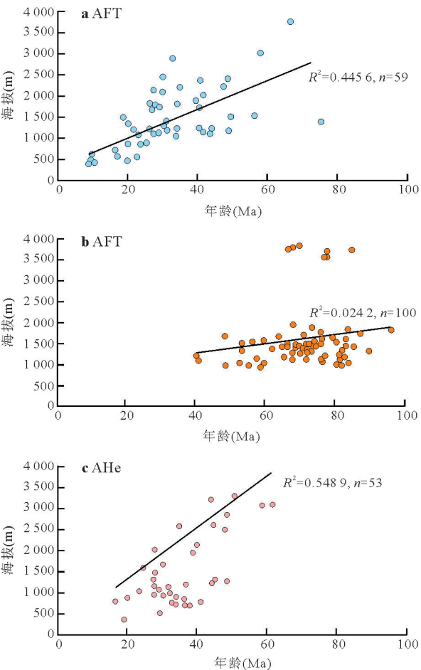
图5 秦岭地区低温热年代学数据年龄—海拔散点图 Fig. 5 Age-altitude scatter plot of low-temperature thermochronological data a. 东秦岭地区低温热年代学 AFT 数据; b. 西秦岭地区低温热年代学 AFT 数据; c. 西秦岭地区低温热年代学 AHe 数据; R^2 . 趋势线拟合程度的指标
