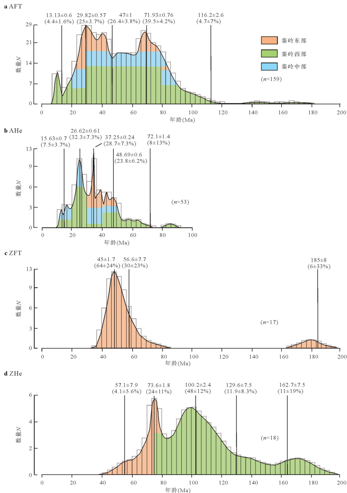
图2 秦岭北麓及周边地区部分已发表的低温热年代学数据分布
