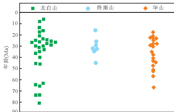
图 3 太白山与华山磷灰石裂变径迹及终南山磷灰石(U-Th)/He 年龄分布
