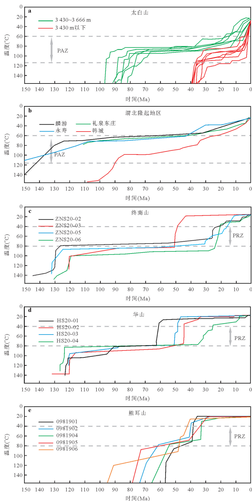
图4 秦岭地区热史反演模拟
