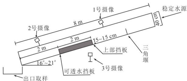
图1 实验水槽及泥沙堆积物布置
