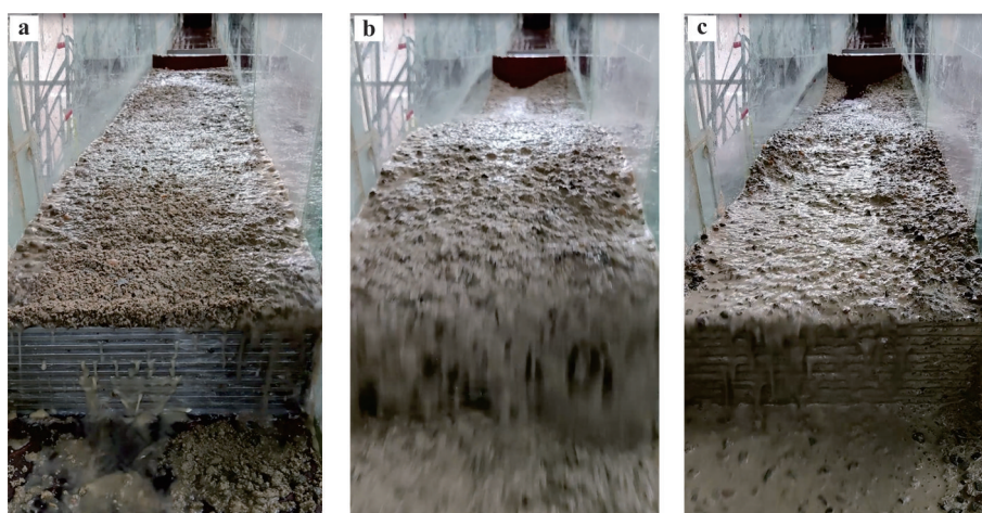
图 7 从下游观测到泥石流起动(第 8 次实验)
