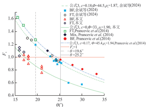
图9 稳定系数与底床坡度关系
