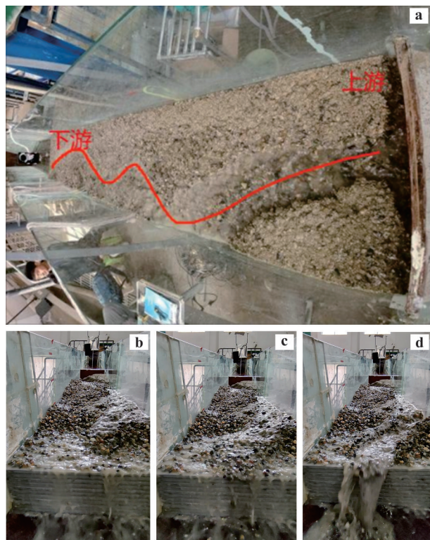
图3 河流运输模式泥石流(第2次实验)
