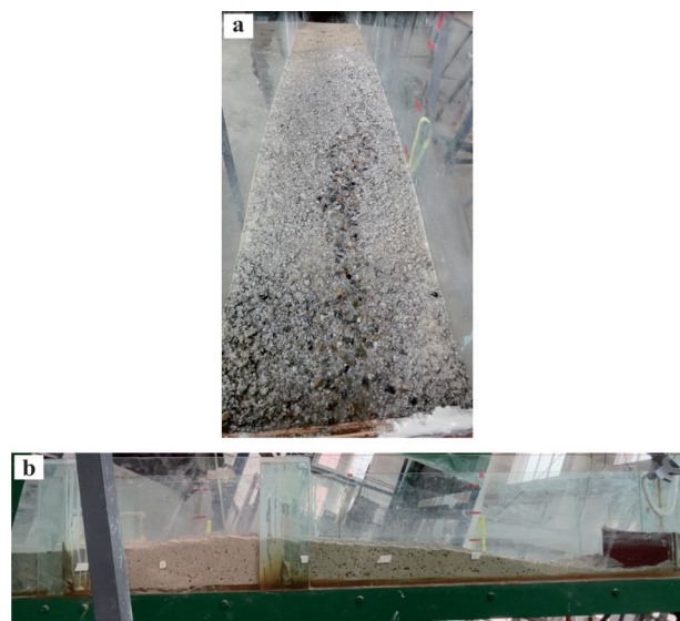
图8 底床失稳模式的泥石流起动(第14次实验)
