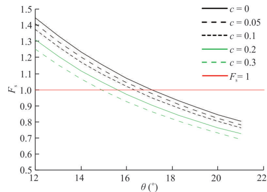
图 13 不同表面流深度下的底坡坡度与稳定系数关系
