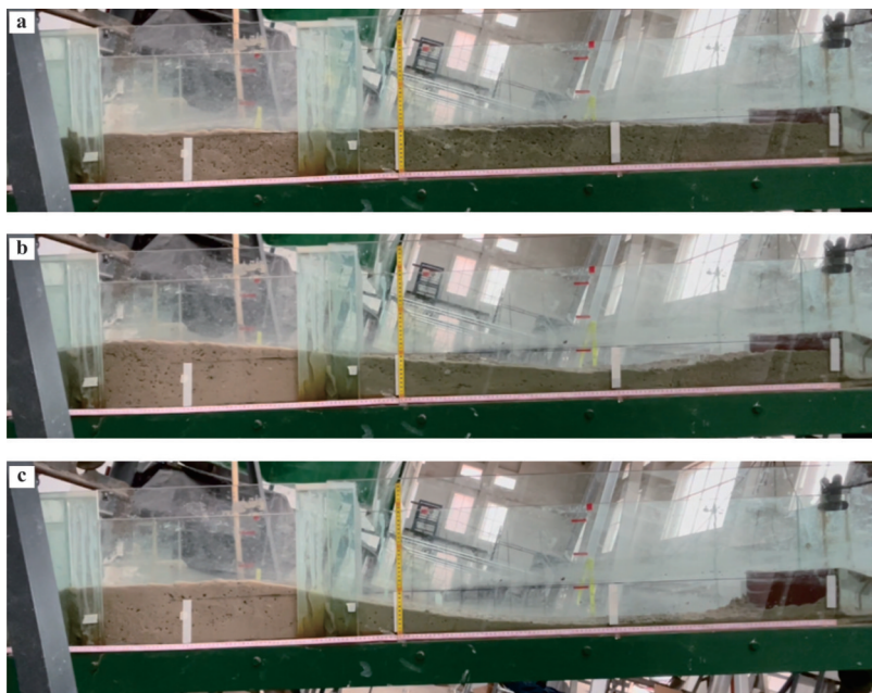
图 6 侧壁观测泥石流起动过程(第 8 次实验)
