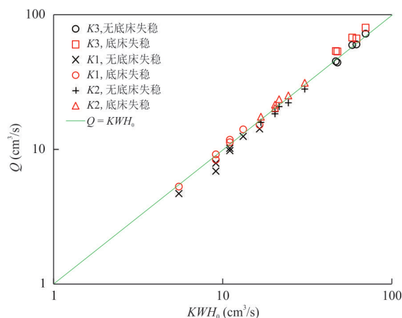
图11 流量与渗透系数、水槽宽度、饱和深度之积的关系
