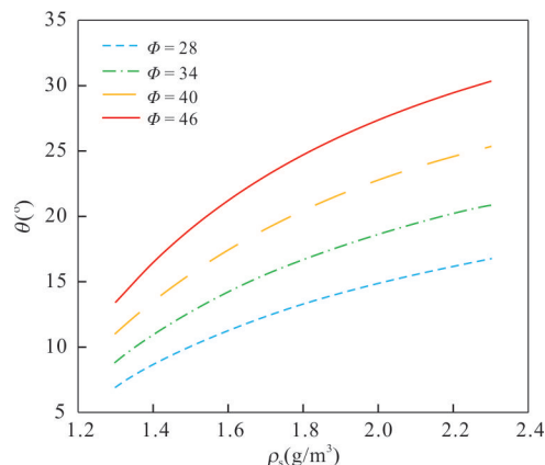
图10 不同内摩擦角条件下的阈值坡度与饱和密度关系
