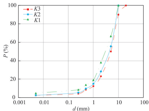
图2 泥沙堆积物粒径分布
