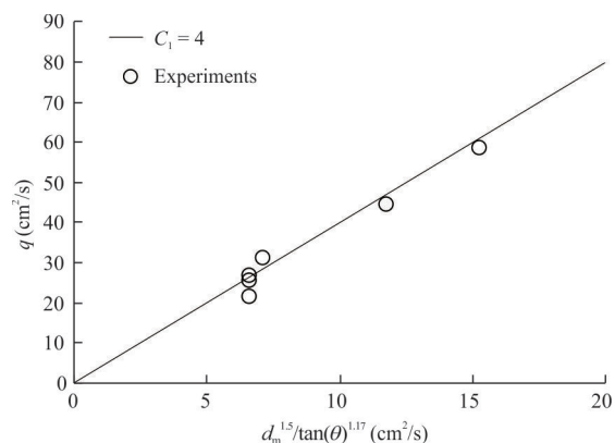
图 12 河流输运模式临界流量与中值粒径和底坡坡度关系
