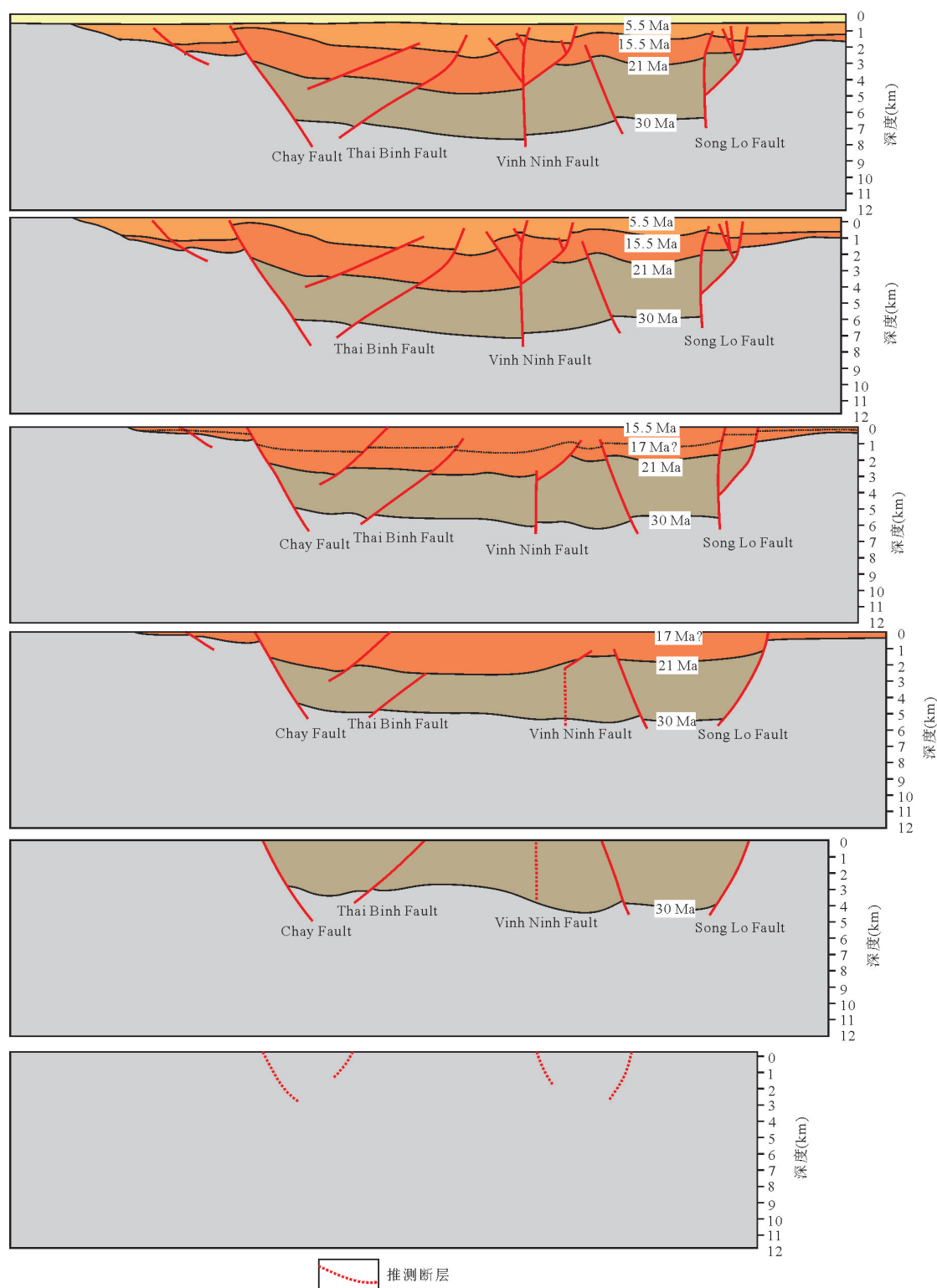
图7 河内凹陷海域区Chay断层、Thai Binh断层、Vinh Ninh断层及Song Lo断层构造演化(剖面位置见图1的4号线)
