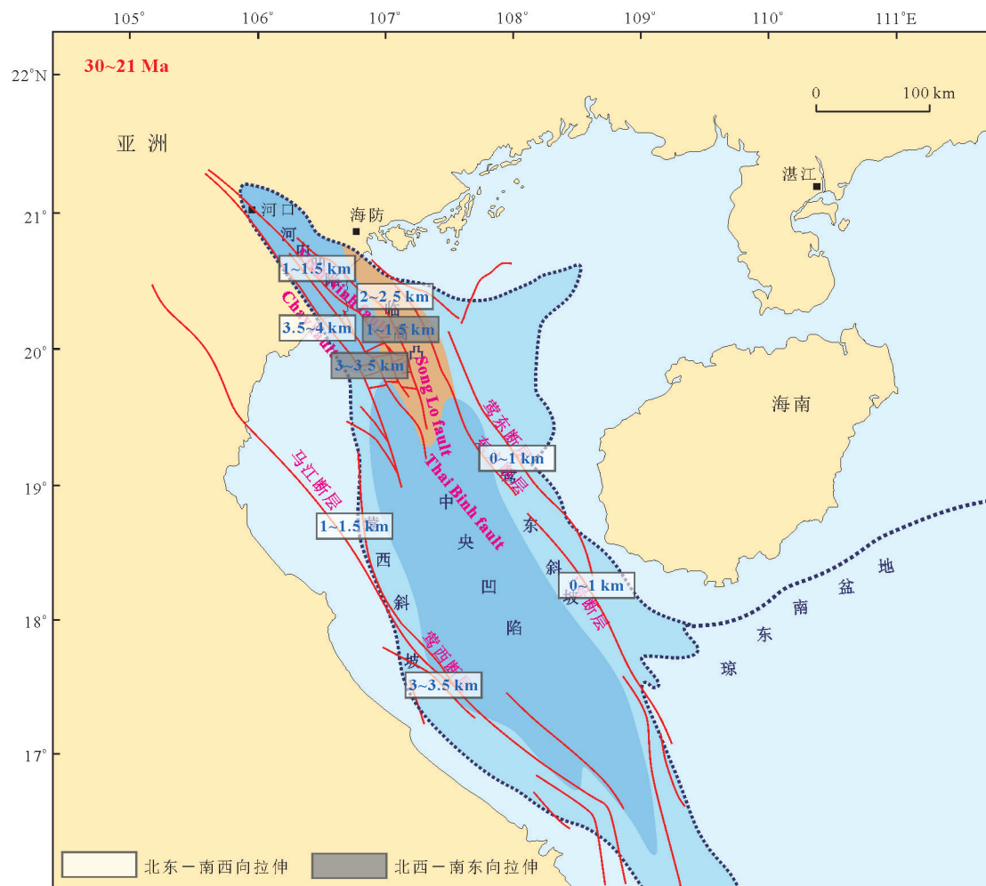
图 10 30~21 Ma 莺歌海盆地伸展量
