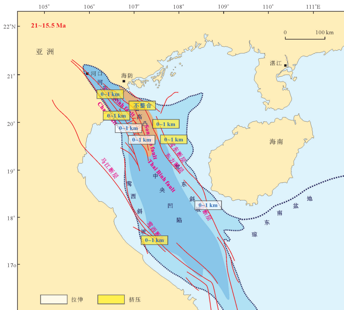
图 12 21~15.5 Ma 莺歌海盆地各个断裂的挤压量
