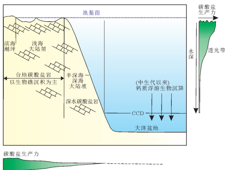
图3 碳酸盐岩沉积环境示意图
