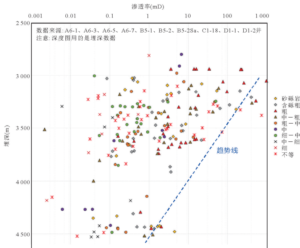
图4 惠州26洼恩平组实测渗透率与埋深关系散点图
