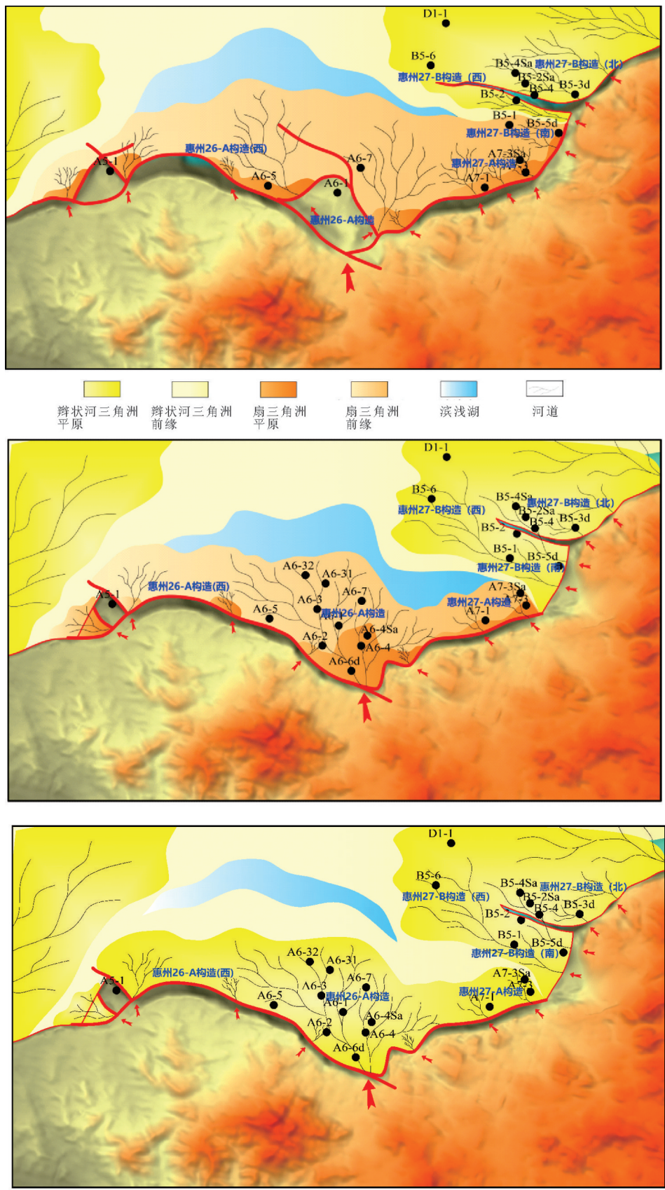
图 3 惠州 26 注恩平组恩三四段沉积相(a)、恩二段早期沉积相(b)、恩二段晚期沉积相(c)
