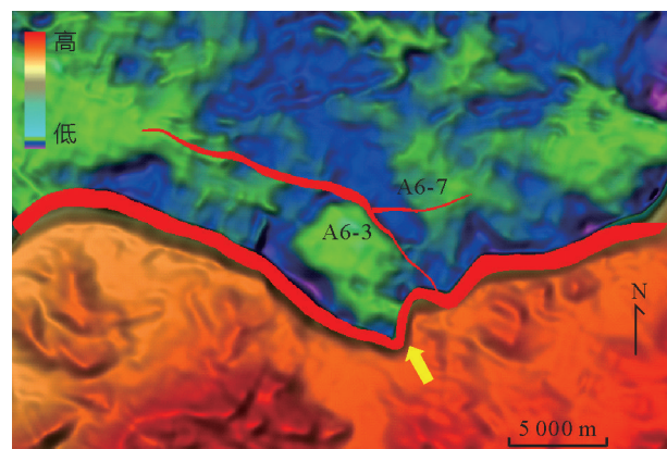
图8 惠州26-A构造EP23层沉积古地貌图(位置见图1b)
