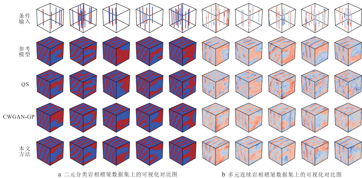
图 10 三维数据集上的可视化对比图
