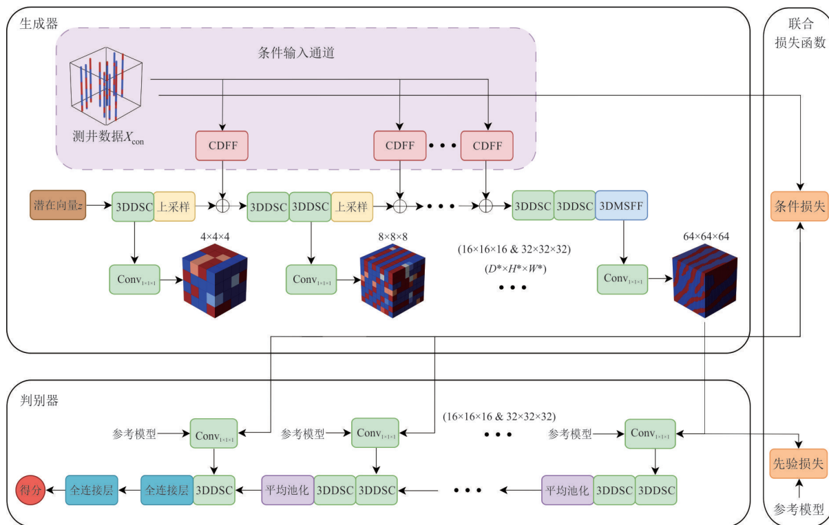
图 1 基于多尺度特征融合和深度可分离卷积的生成对抗网络地质建模方法总体框架设计
