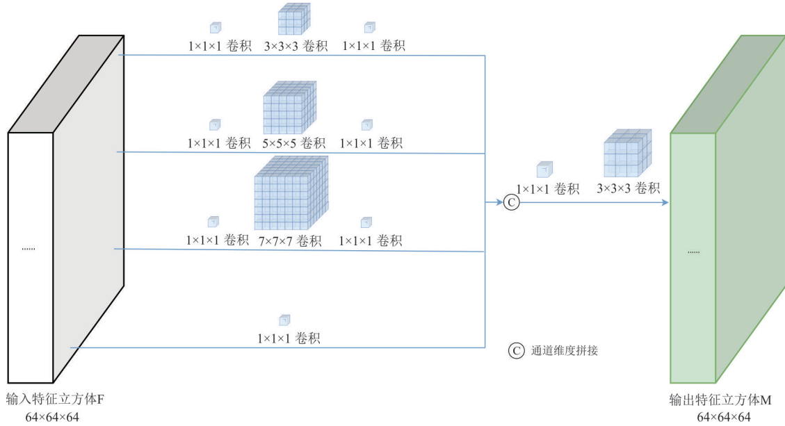
图3 三维多尺度特征融合模块结构图
