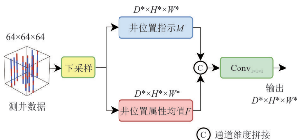
图 2 条件数据特征融合模块结构
