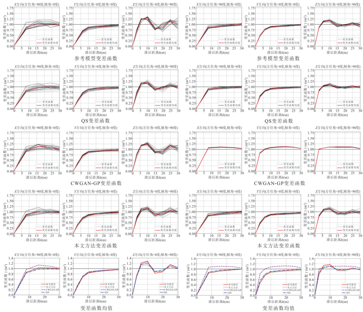
a 二元分类岩相褶皱数据集上的变差函数
