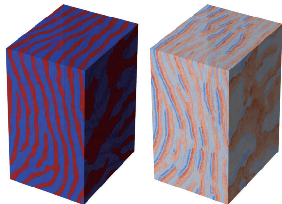
a 二元分类岩相褶皱数据 b 多元连续岩相褶皱数据
