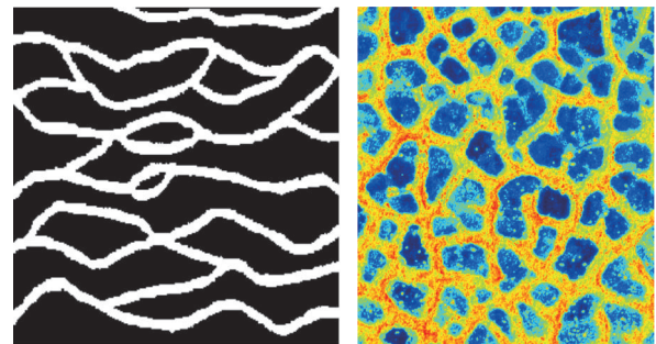
a 二元分类河流相数据 b 多元连续冰楔数据
