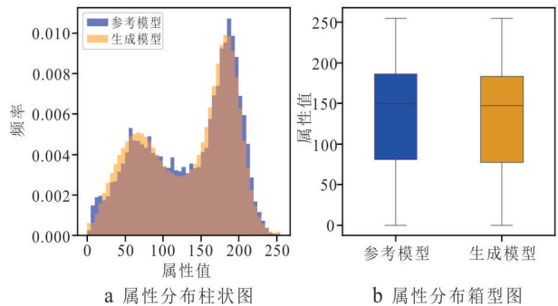
图 8 多元连续冰楔数据集的属性分布柱状图和箱型图
