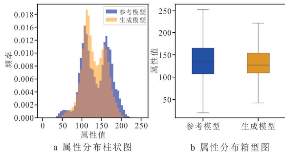
图 12 多元连续岩相褶皱数据集的属性分布柱状图(a)和箱型图(b)
