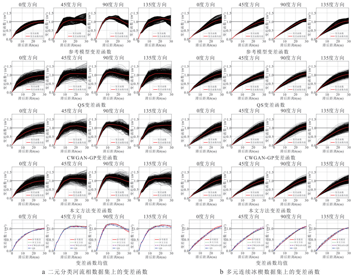
图 7 二维数据集上的变差函数及其均值对比图
