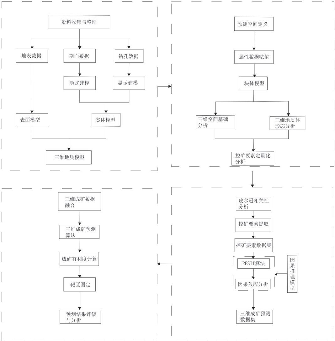
图3 研究技术路线 Fig.3 Research and technology road map
