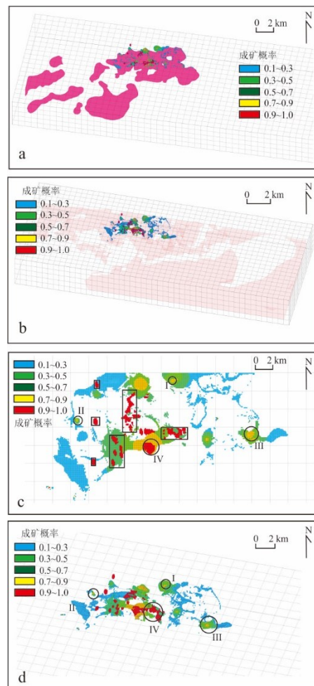
图14 三维成矿预测靶区图
