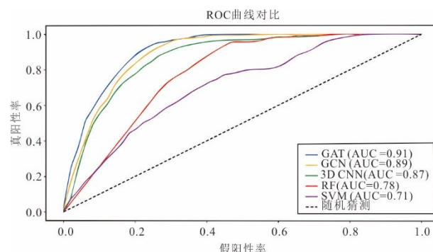
图10 ROC 曲线效果
