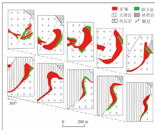
图2 安庆铜矿主矿体剖面示意图
