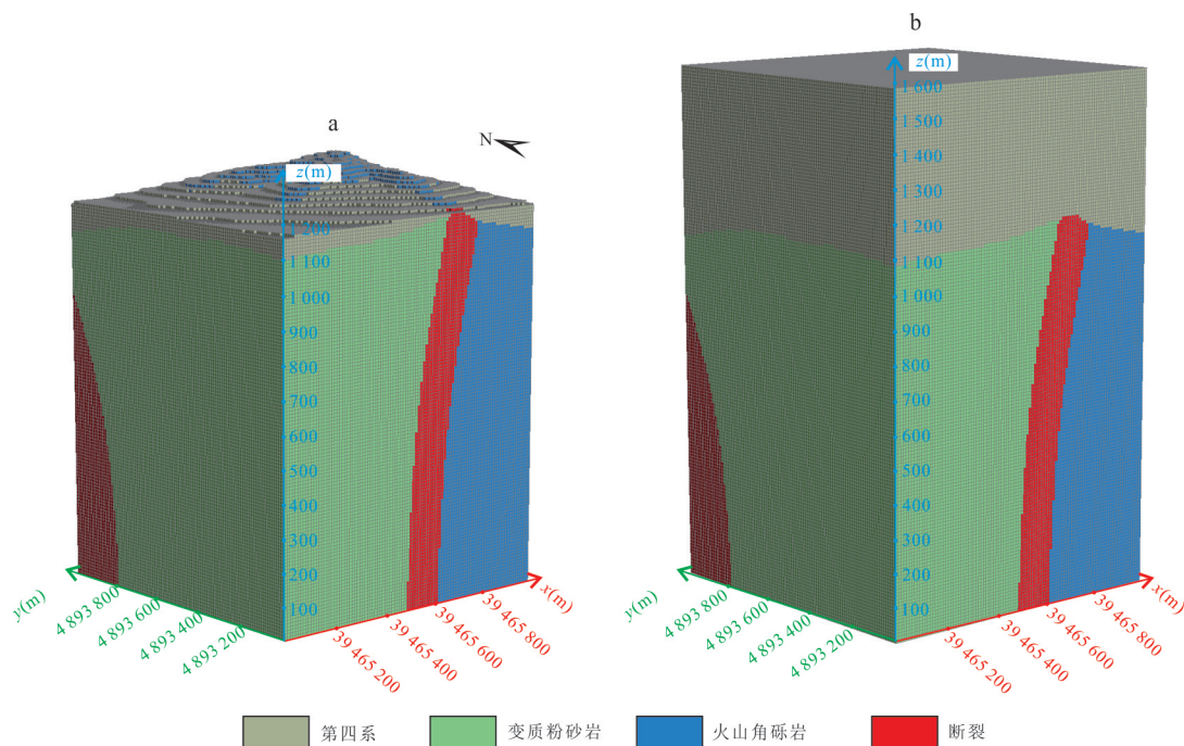
图7 毛登矿区 Flac 3D 六面体模型
