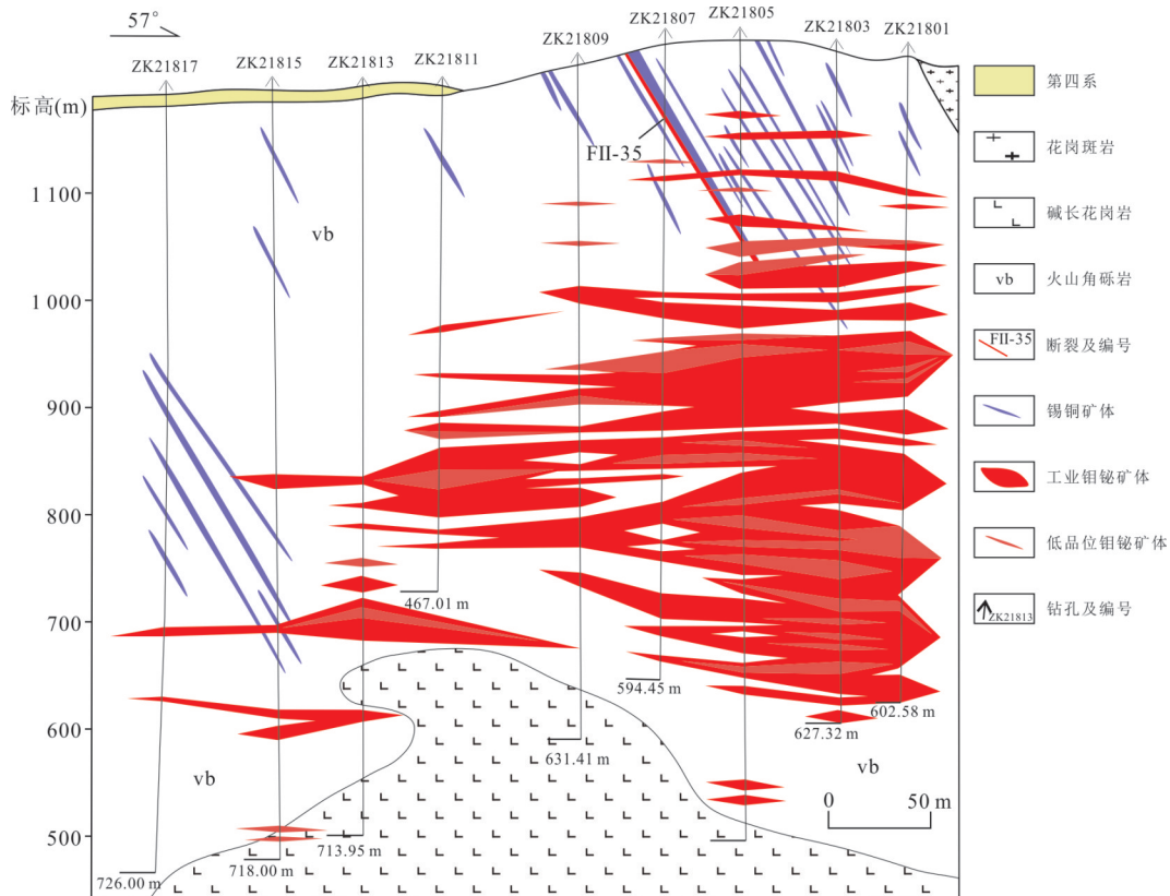
图14 毛登矿床218号勘探线剖面(据季根源等, 2022修改)
