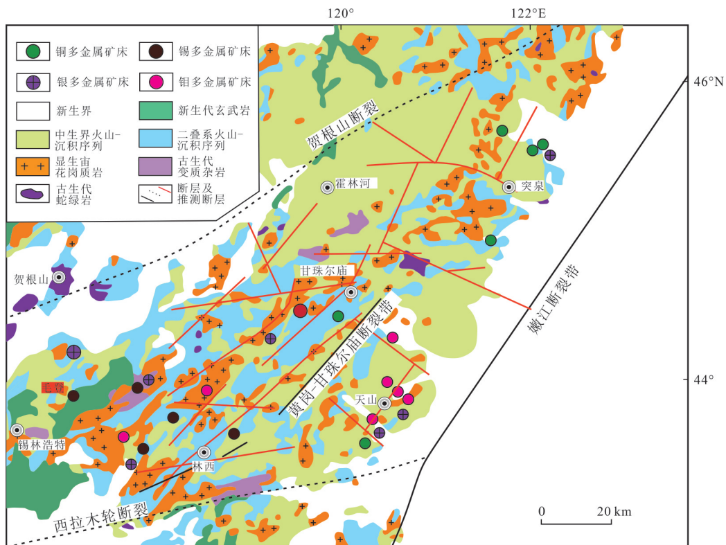
图1 大兴安岭南段地质简图及矿床分布(据Li et al. , 2024)
