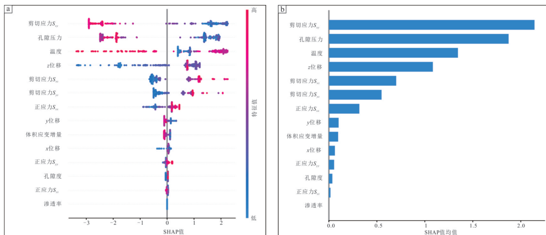
图 10 SHAP 解释图
