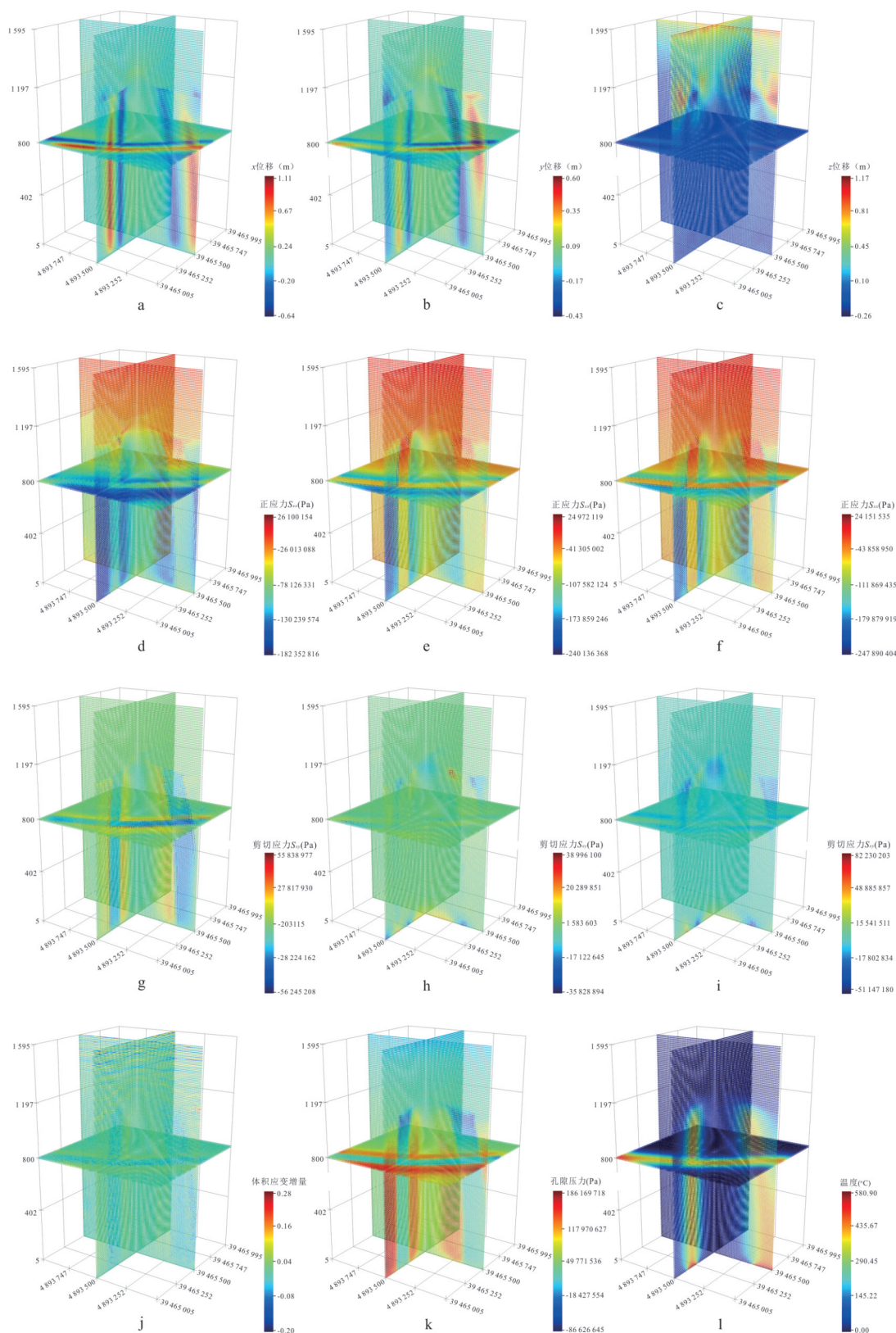
图8 Flac 3D 模拟结果各条件三维可视化图
