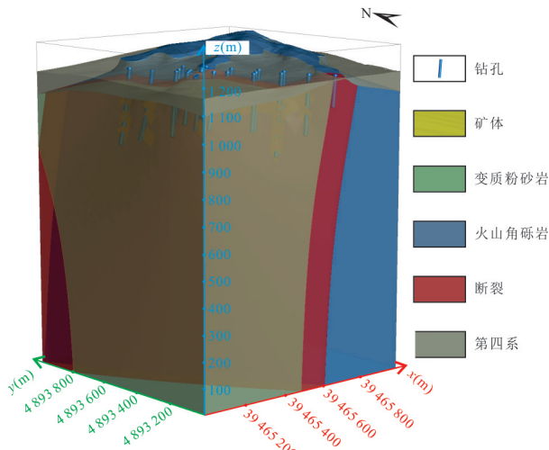
图 6 研究区三维地质模型
