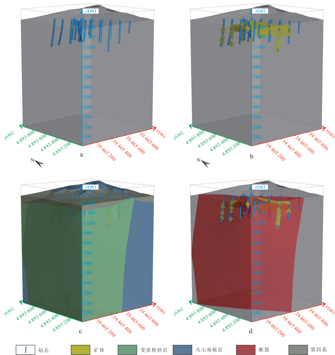
图 4 毛登矿区三维地质模型
