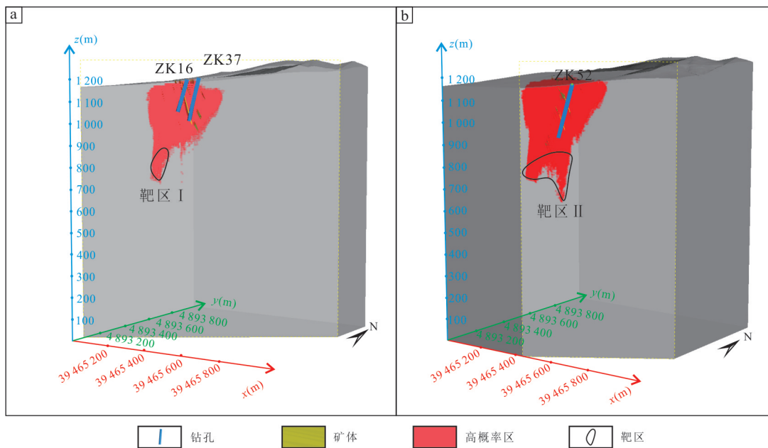
图 13 剖面靶区示意图
