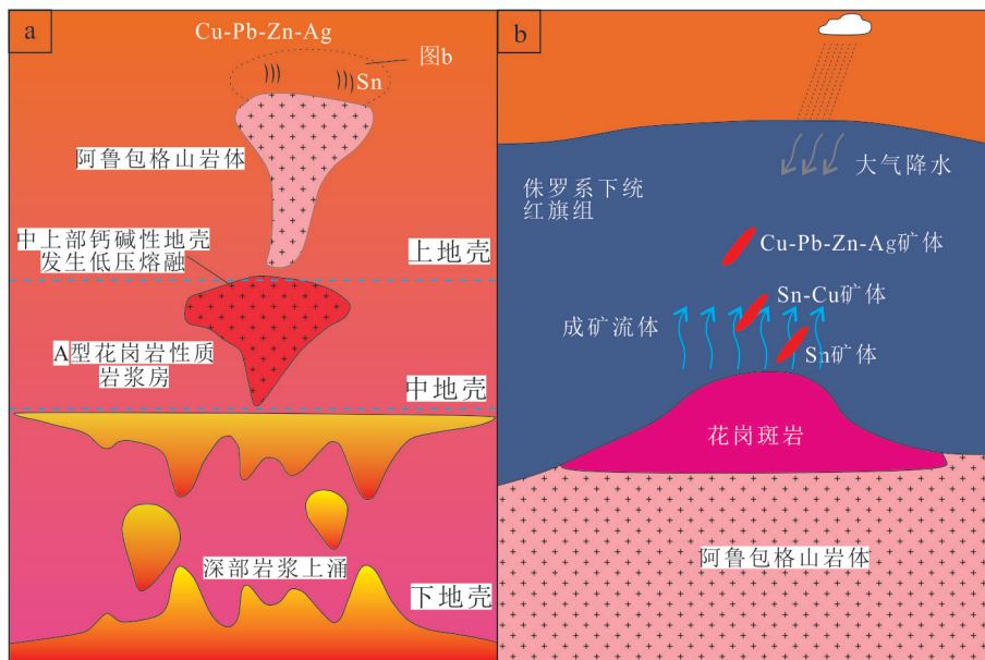
图3 毛登锡铜矿床成矿模式
