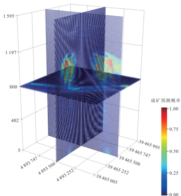
图 11 毛登矿区成矿概率
