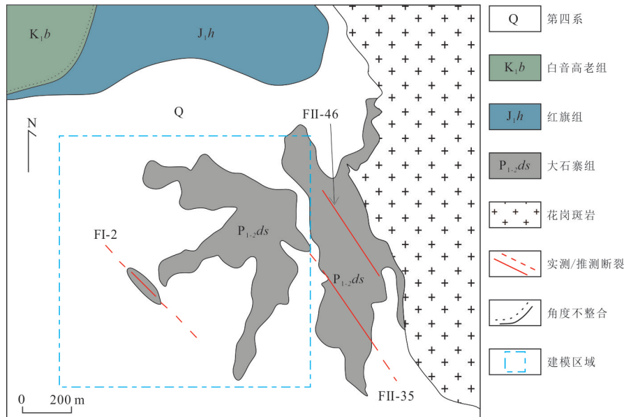
图2 毛登 Sn-Cu 矿床地质简图(据季根源等, 2021b 修改)
