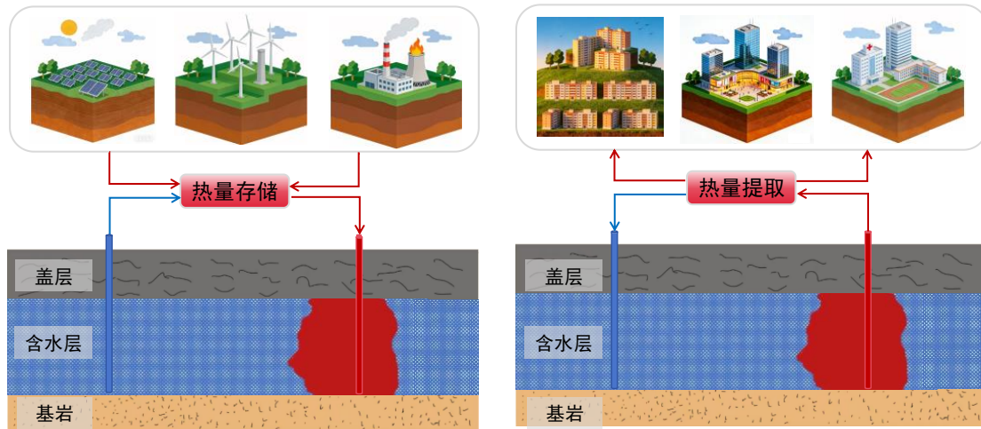
图4 含水层储能系统示意(黄永辉等, 2023; Geerts et al. , 2025)
