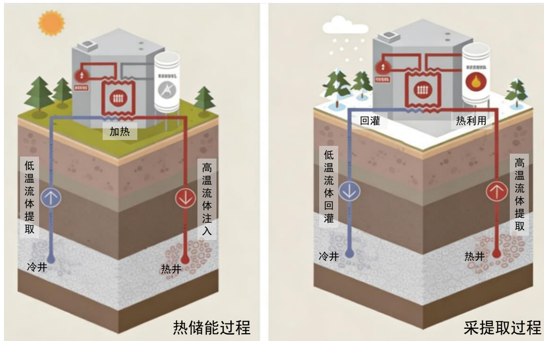
图1 深部地热储能示意(黄永辉等,2020)
