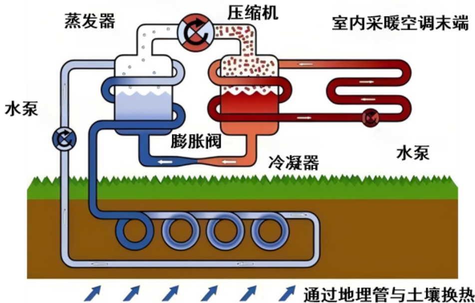
图 5 岩土储能系统示意( https://wenku.baidu.com )
