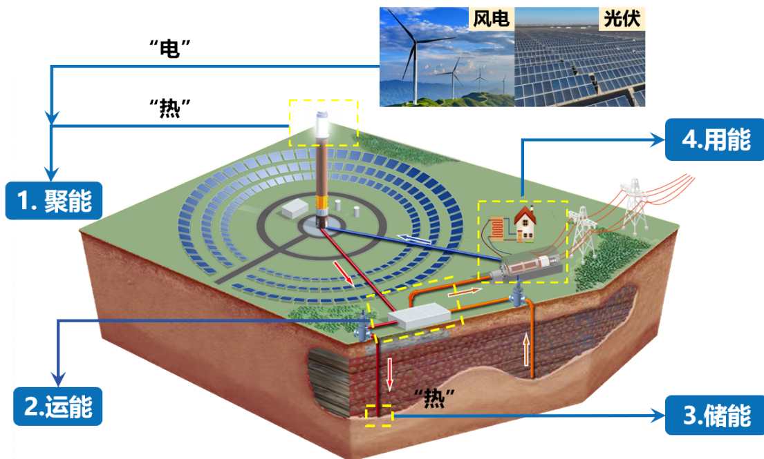
图8 “地大方案”——地下超长时高温储能系统概念
