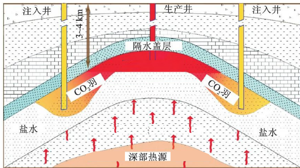
图7 二氧化碳羽流储能示意(周倩等, 2023)
