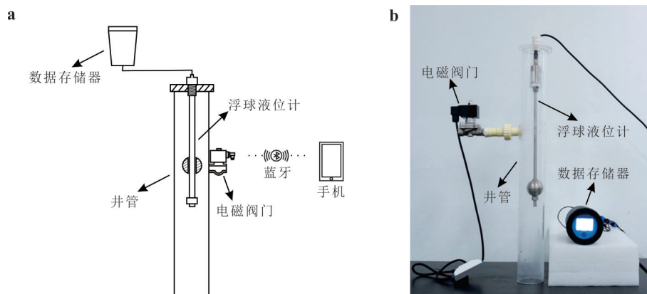
图1 自动渗流仪
