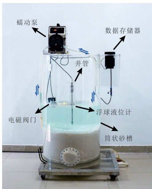
图4 地下水—地表水交换通量试验装置
