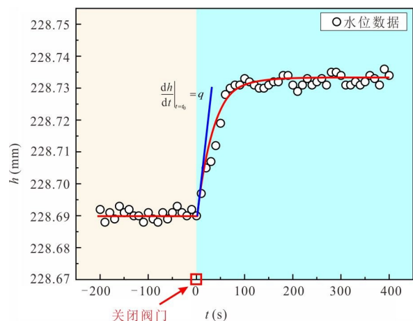
图10 野外监测水位—时间动态曲线
