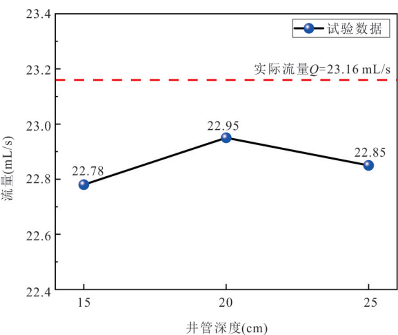
图 8 自动渗流仪流量与实际流量对比 Fig.8 Comparison of automatic seepage meter flow and actual flow
