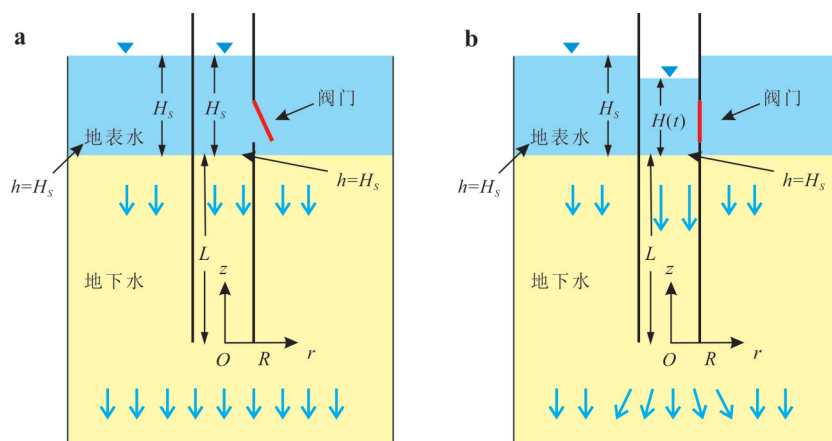
图2 地下水—地表水交换通量监测评估原理(据 Zlotnik et al. , 2023 修改)
