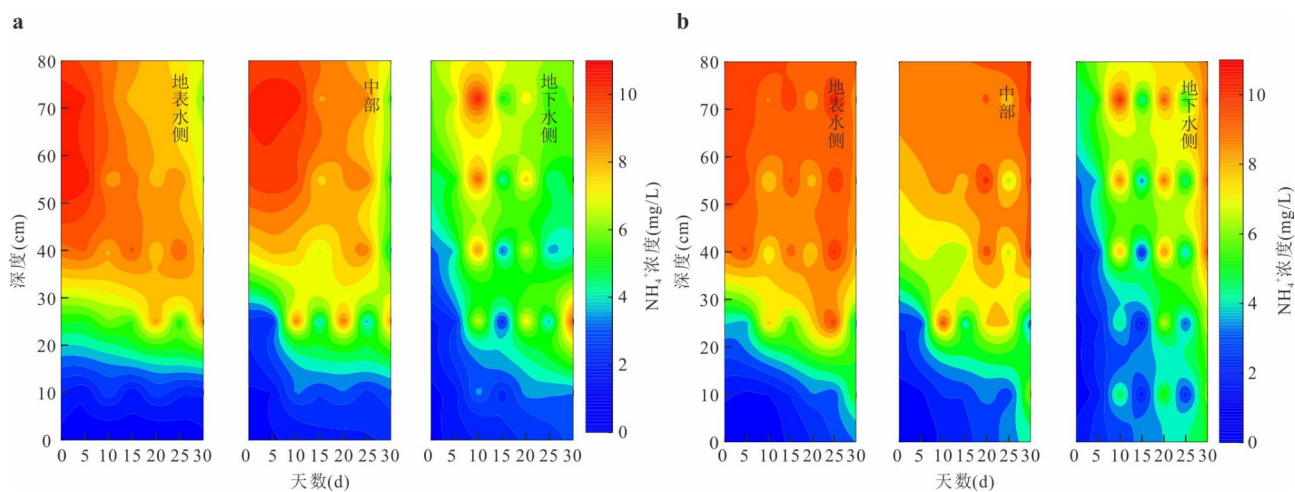
图4 不同水力梯度下沉积物孔隙水 \text{NH}_4^+ 变化特征
