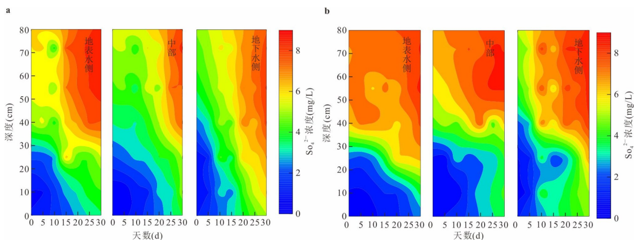
图5 不同水力梯度下沉积物孔隙水 \text{SO}_4^{2-} 变化特征
