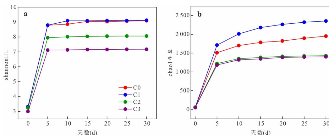
图6 潜流带沉积物样品 Shannon 指数稀释曲线(a)和 Chao1 指数(b)
