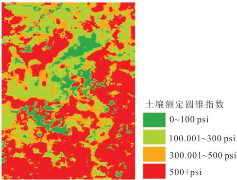
图 4 土壤额定圆锥指数 Fig.4 Soil rating cone index (RCI) distribution
