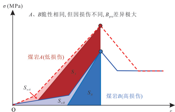
图1 同脆性异损伤煤岩应力-应变对比
