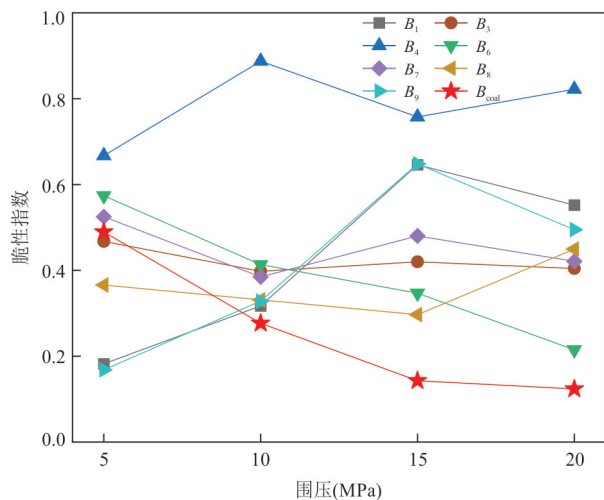
图 12 不同围压条件下煤岩的脆性指标评价结果
