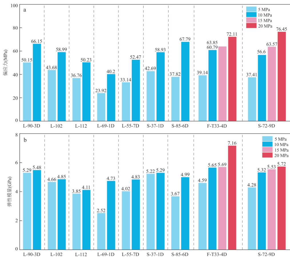
图 11 不同围压下煤岩力学参数
