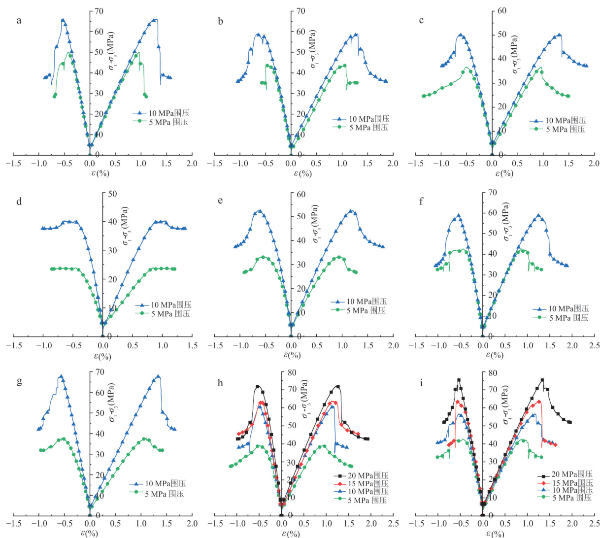
图10 不同围压下应力应变曲线
