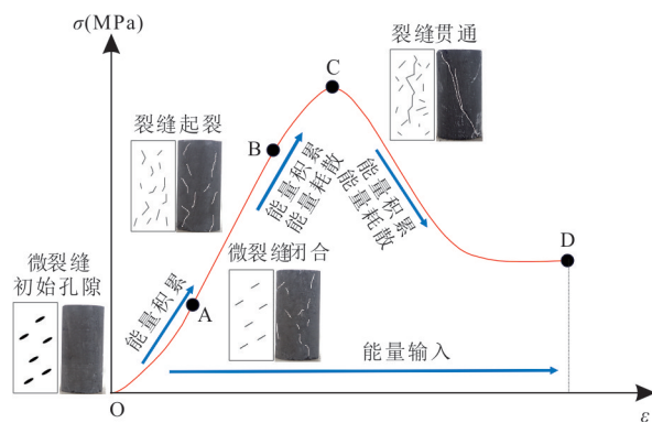
图9 岩石应力-应变曲线及能量转化示意图
