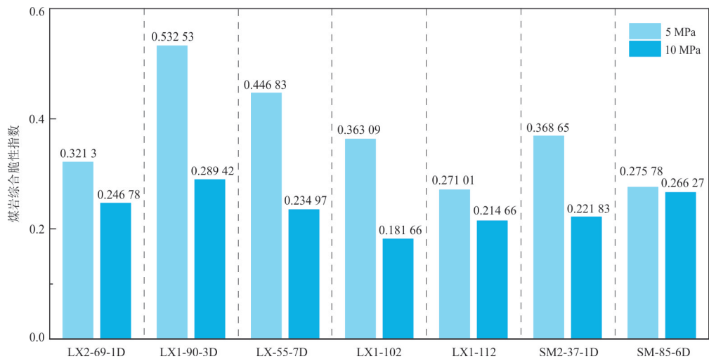
图 14 不同围压下 7 组煤岩的脆性指数
