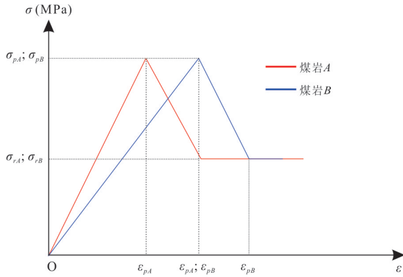
图2 脆性指标 B_7 、 B_8 未能反映的情况
