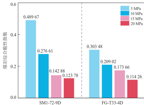
图 13 不同围压下两组煤岩的脆性指数对比
