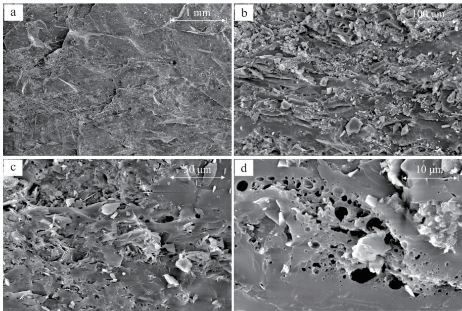
图3 煤岩微观结构扫描电镜图 Fig. 3 Scanning electron microscope images of coal-rock microstructure a. 放大100倍;b. 放大1 000倍;c. 放大2 000倍;d. 放大10 000倍
