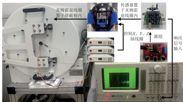
图4 性能测试平台实物图
