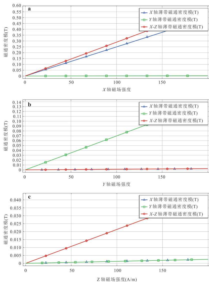
图 2 (a)X 方向磁场下各探头敏感材料磁通密度变化;(b)Y 方向磁场下各探头敏感材料磁通密度变化;(c)Z 方向磁场下各探头敏感材料磁通密度变化
