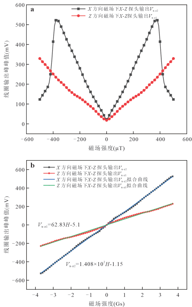
图6 (a)X-Z轴探头输出 V_{x-z1} 和 V_{x-z2} ; (b) \pm 370 \mu T 范围内 X-Z 轴探头输出 V_{x-z1} 、 V_{x-z2} 的响应曲线及拟合曲线
