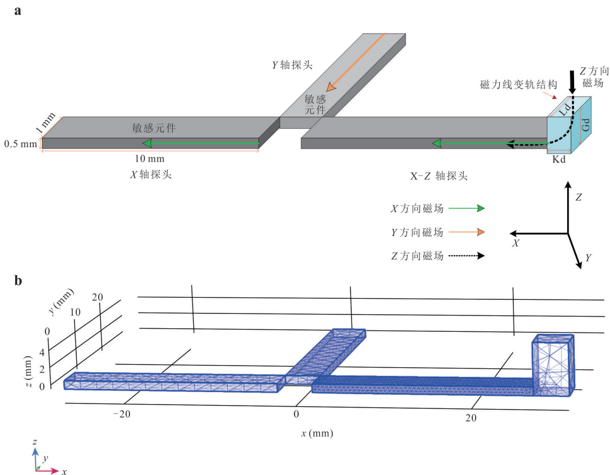
图1 (a)平面三轴GMI磁传感器三轴磁探头的模型构建图;(b)网格剖分图
