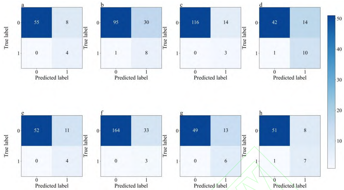
图 3 模型在测试集上推理结果的混淆矩阵
