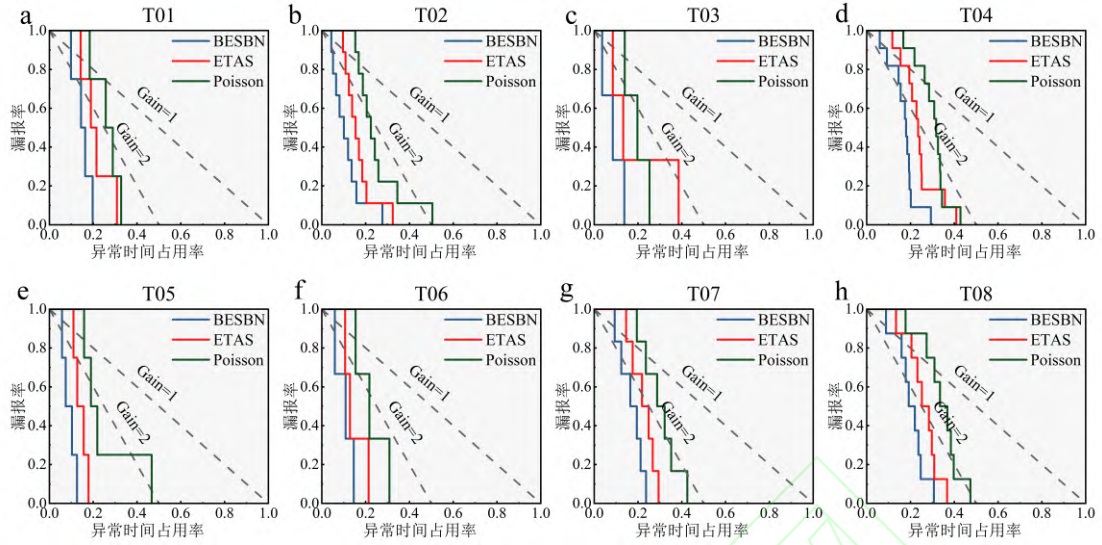
图 7 不同区域模型的 Molchan 图
