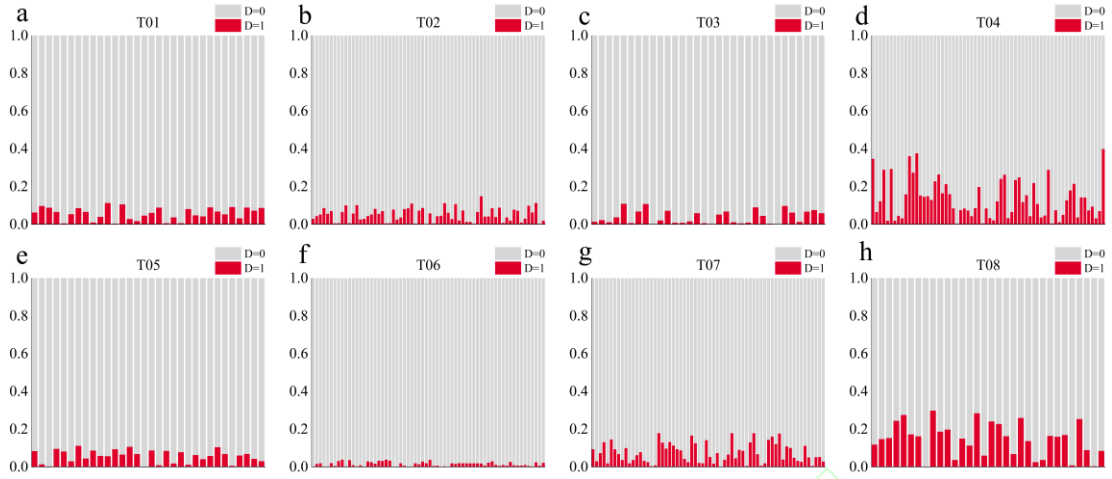
图 6 8 个区域中 BESBN 的条件概率表
