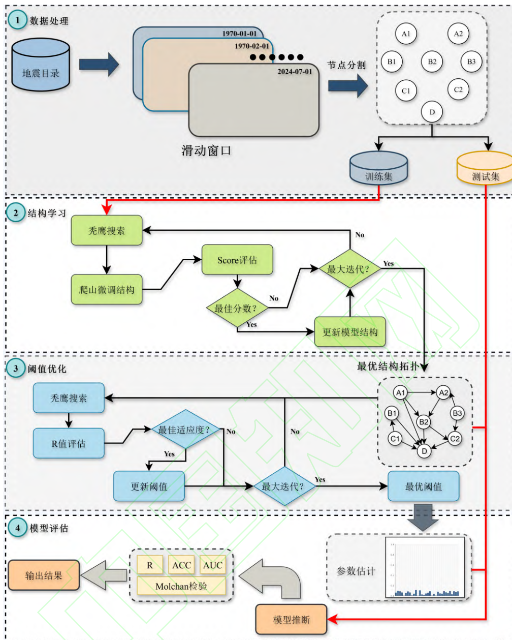
图 2 研究方法的框架与流程
