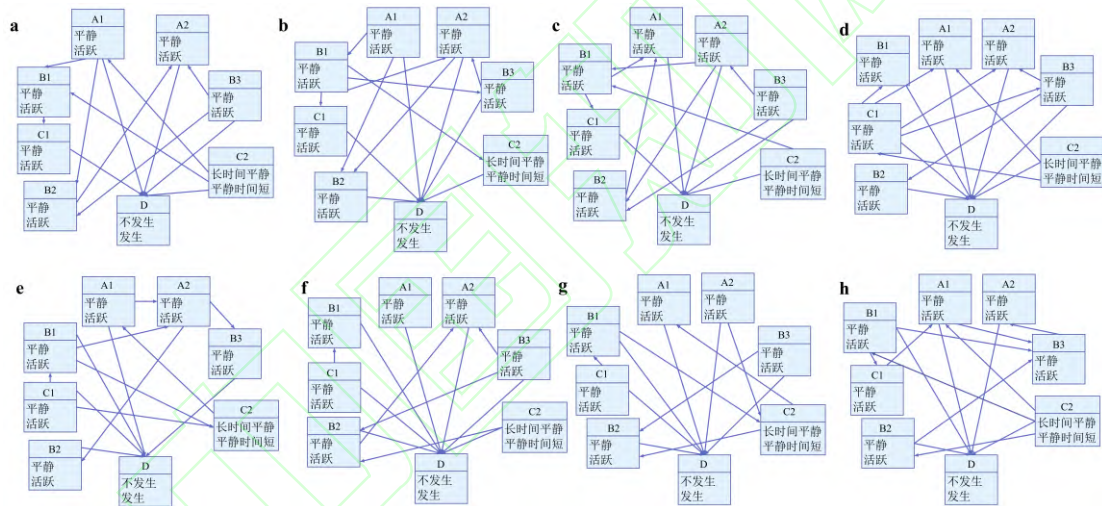
图 4 不同区域的 BESBN 网络结构对比
