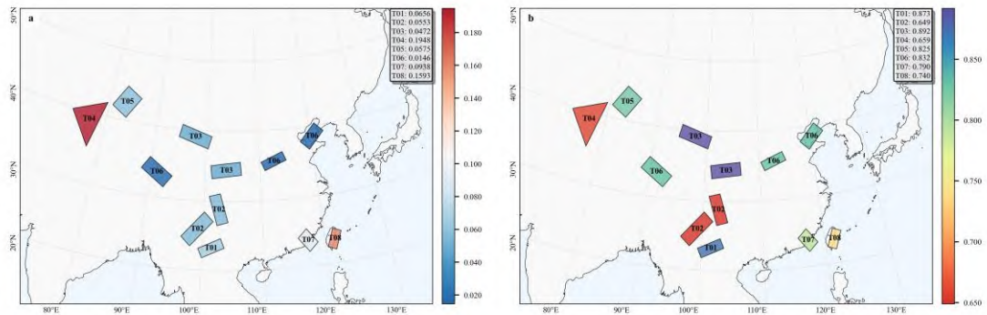
图 5 8 个区域的 BESBN 报警阈值与 R 值
