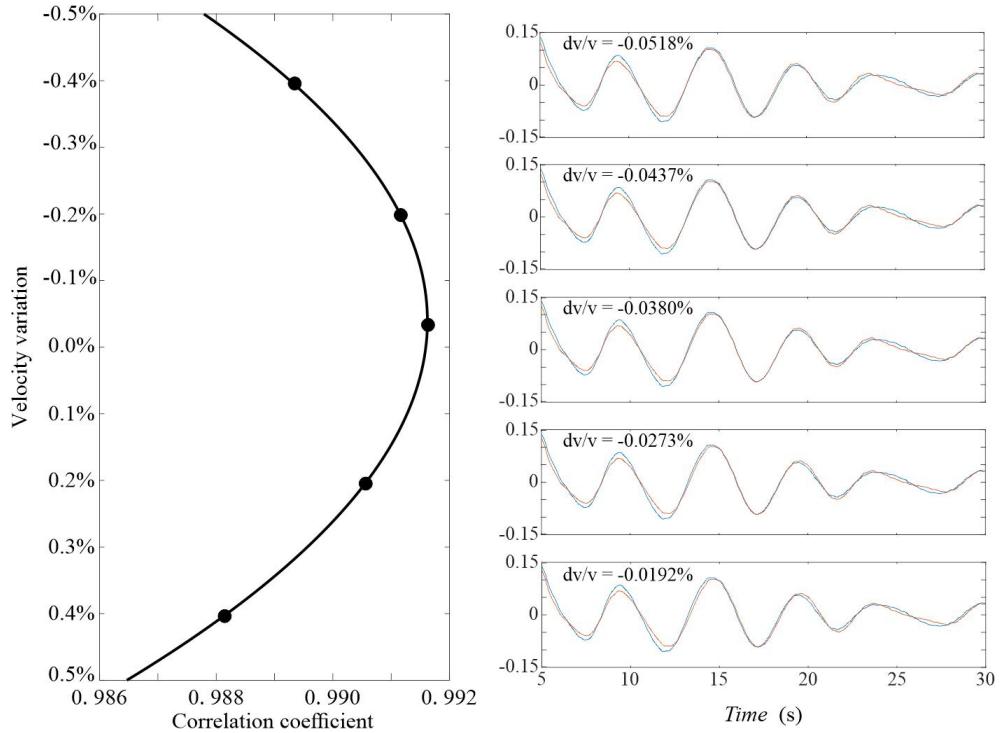
图 4 压缩拉伸法进行波速测量示例
