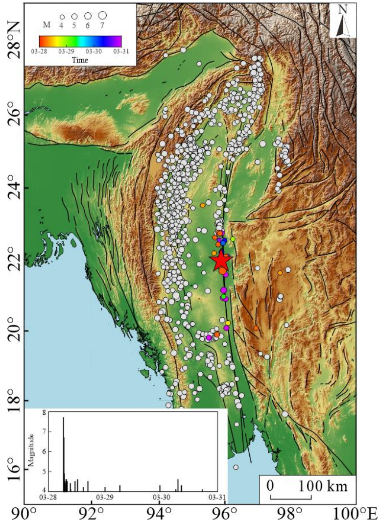
图 2 区域地震活动性
