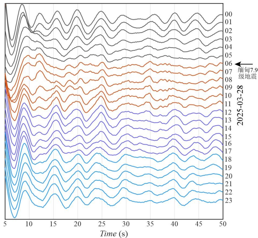
图 7 NGU 台 2025 年 3 月 28 日自相关函数变化
