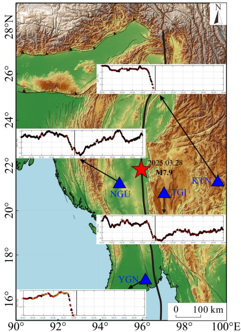
图 8 不同台站在缅甸地震前后的地震波速相对变化(0.1-2 Hz)，其中 KTN 和 YGN 台缅甸地震期间数据缺失。
