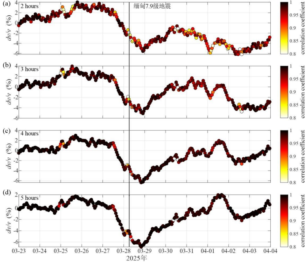
图 6 NGU 台 0.1-2 Hz 频率范围不同滑动窗口的相对波速变化(黑色实线为缅甸地震发震时刻)
