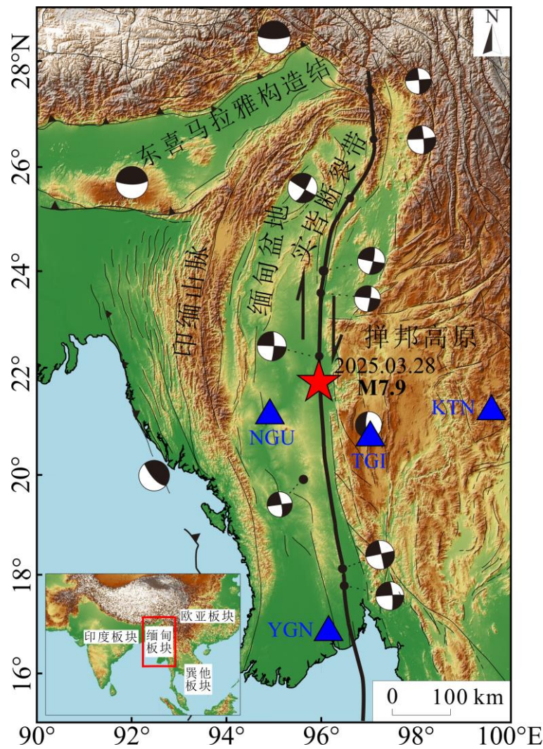
图 1 区域地质构造、台站及历史强震(M>6.5)分布图
