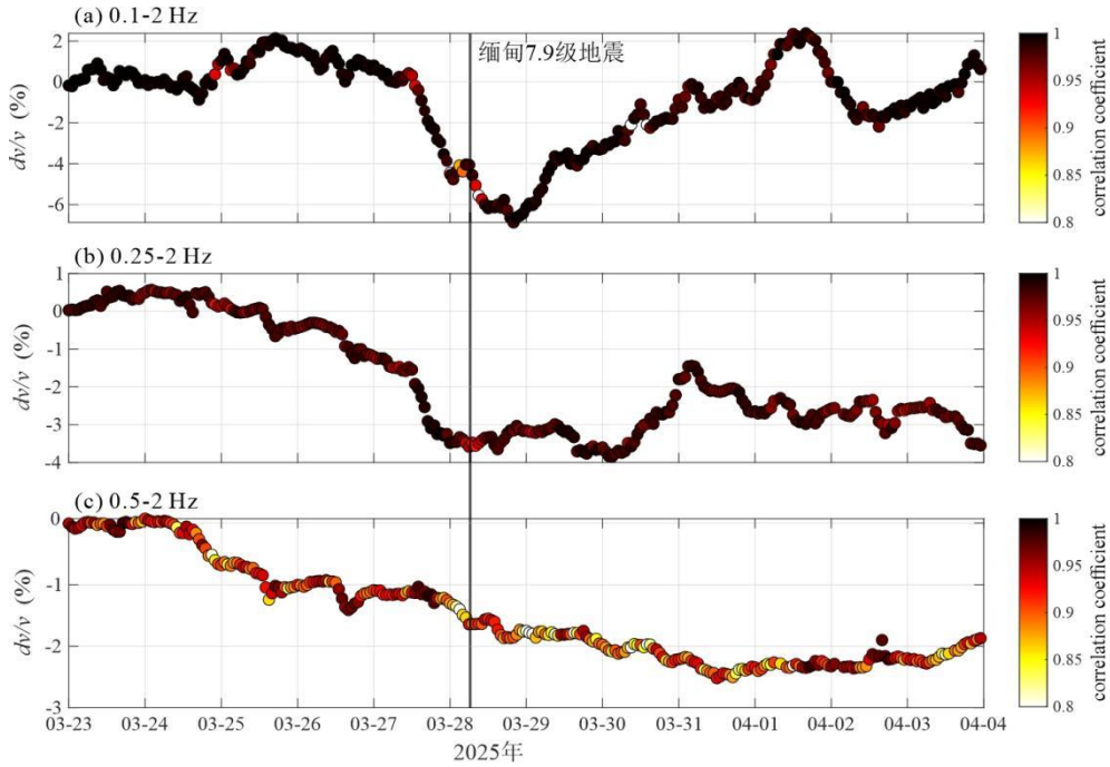
图 5 NGU 台不同频率范围随时间的相对波速变化(黑色实线为缅甸地震发震时刻)
