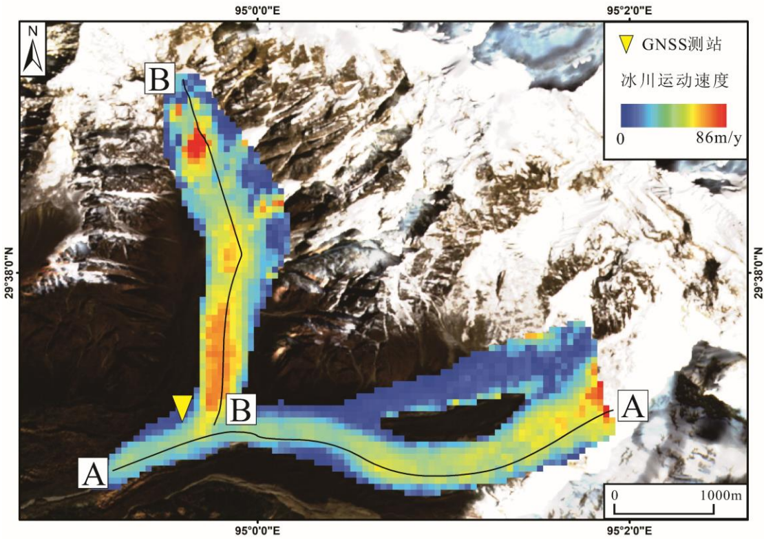
图 6 则隆弄冰川 2022.7-2023.7 平均速度分布差异及 GNSS 测站位置
