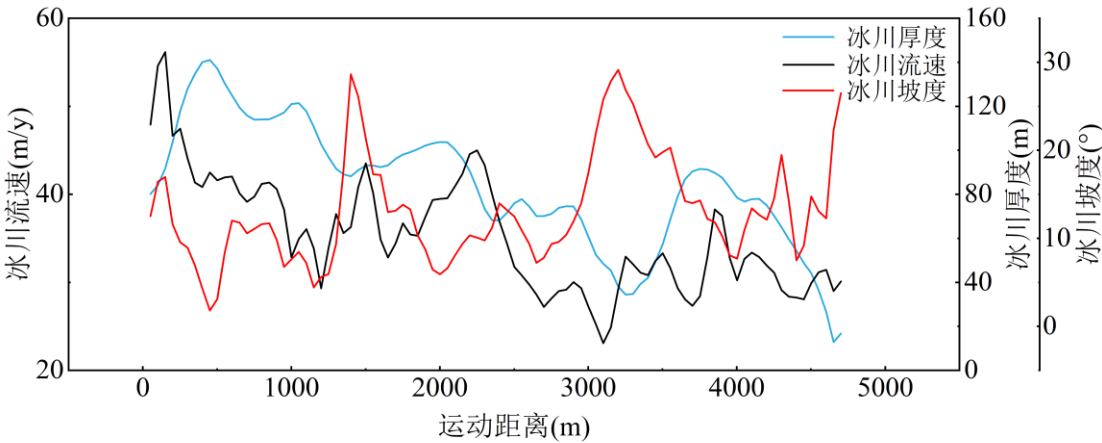
(1) A-A剖面冰川流动速度与坡度和厚度的关系
