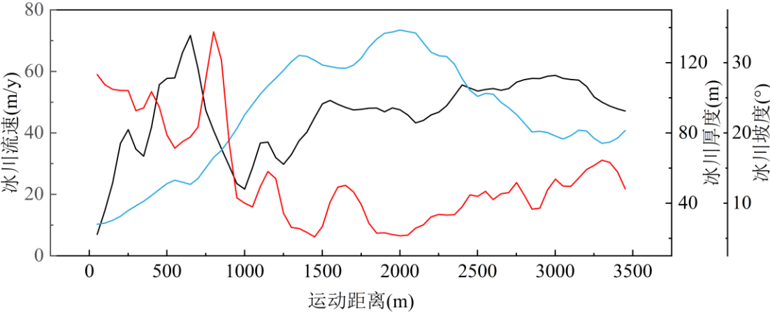
(2) B-B剖面冰川流动速度与坡度和厚度的关系
