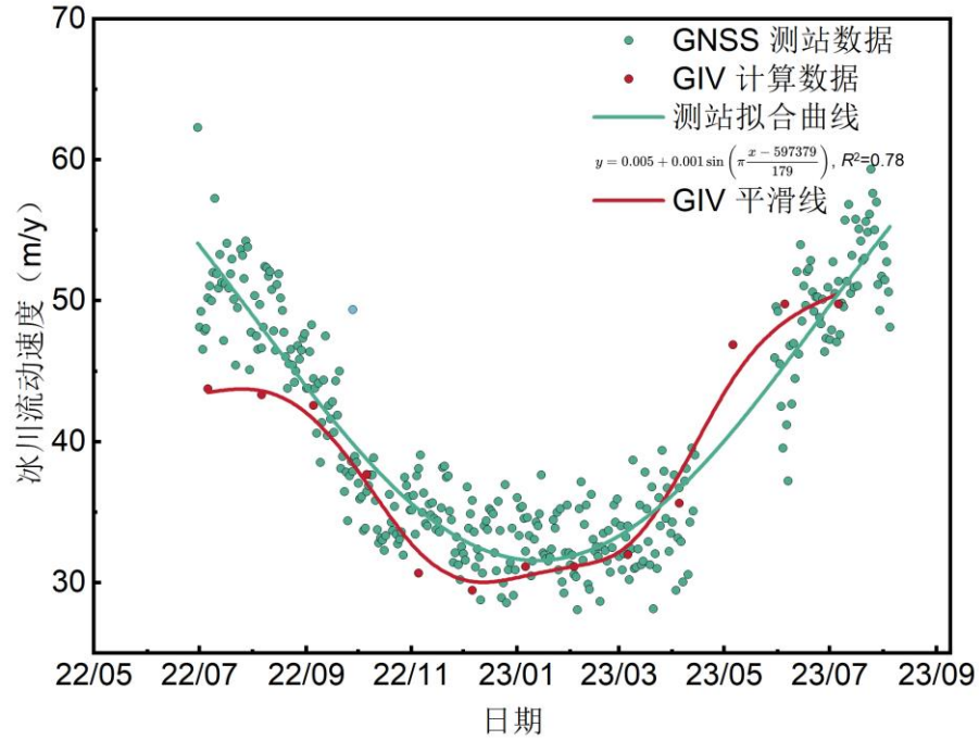
图7 则隆弄冰川流速计算数据与实测数据对比图
