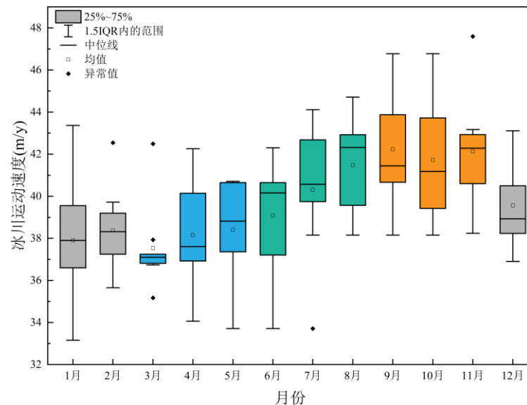
图 5 则隆弄冰川流速季节分布
