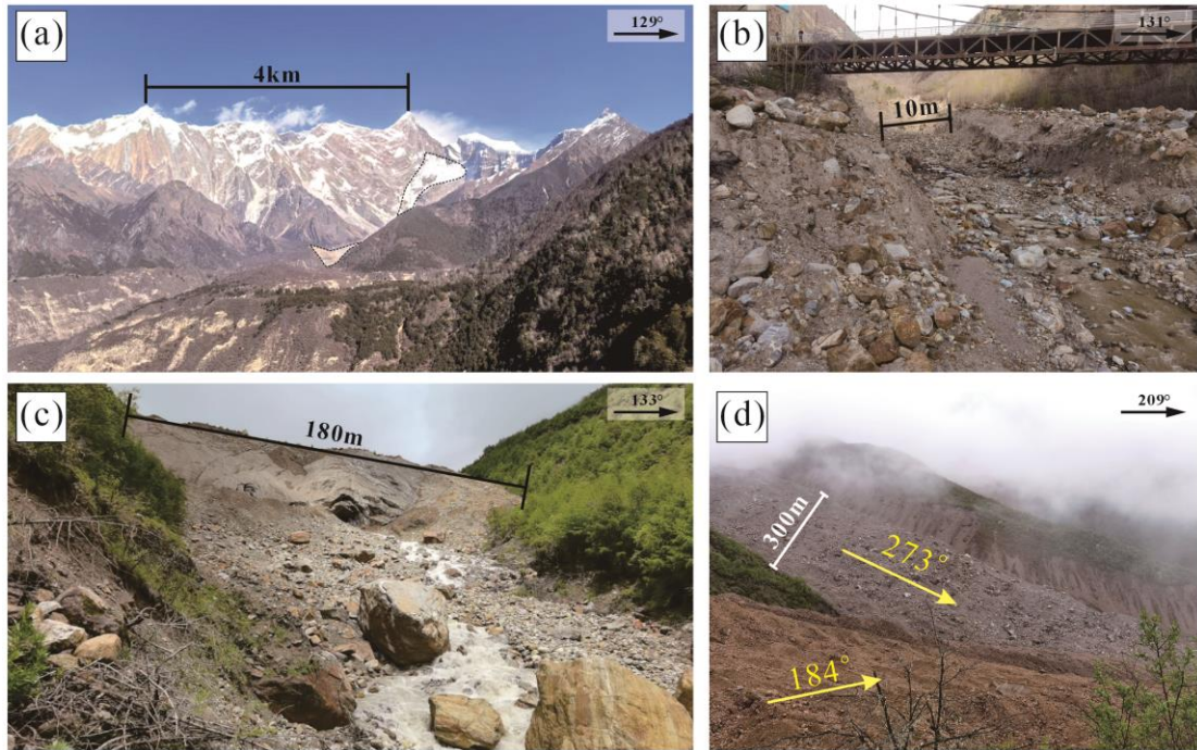
图 2 研究区现场照片 (a) 则隆弄冰川区远景 (b) 直白大桥及下游沟道 (c) 则隆弄冰川冰舌区物源 (d) 则隆弄冰川交汇处表层照片
