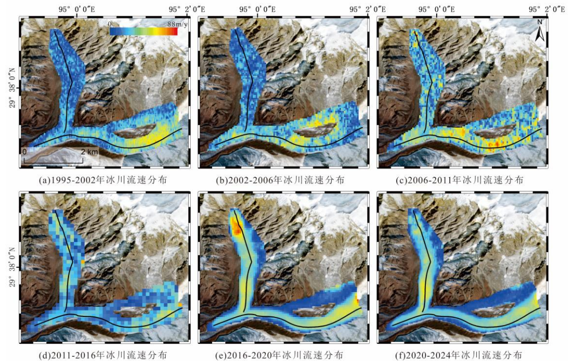
图3 则隆弄冰川不同时期流速图
