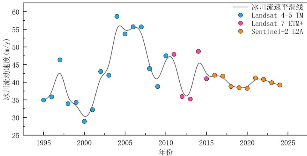
图 4 则隆弄冰川年平均流动速度变化
