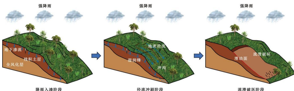
图 4 降雨型浅层滑坡失稳过程示意图（改自冯文凯等，2025）
