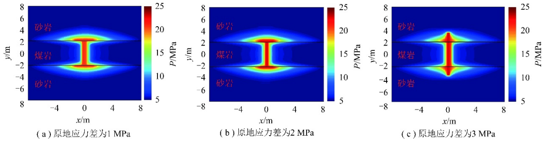
图 6 不同原地应力差条件下裂缝扩展结束时压力云图（据杨兆中等，2021）
