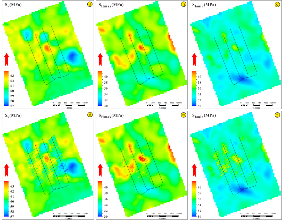
图9 鄂尔多斯盆地东缘佳县地区深部煤层气储层压裂前后地应力分布对比图
