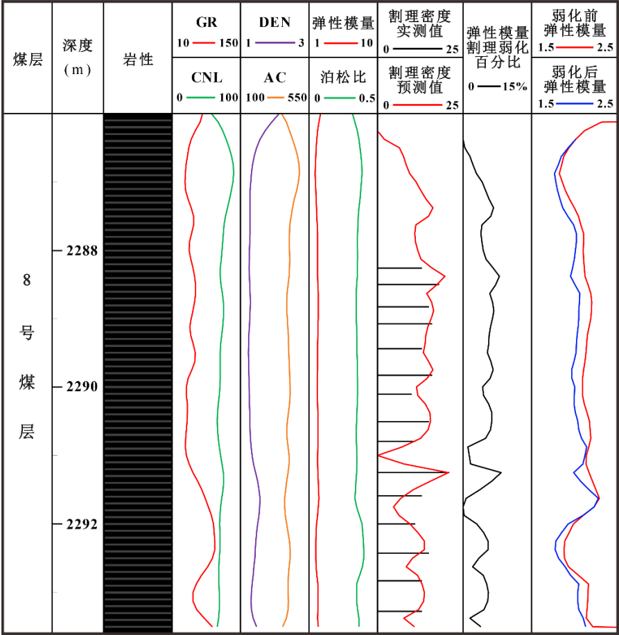
图 7 考虑裂缝弱化效应的鄂尔多斯盆地佳县地区煤层岩石力学剖面图
