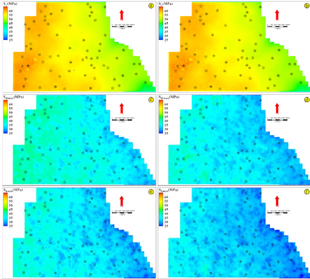
图 8 考虑裂缝影响效应的鄂尔多斯盆地东缘佳县地区深部煤层气储层现今地应力分布图
