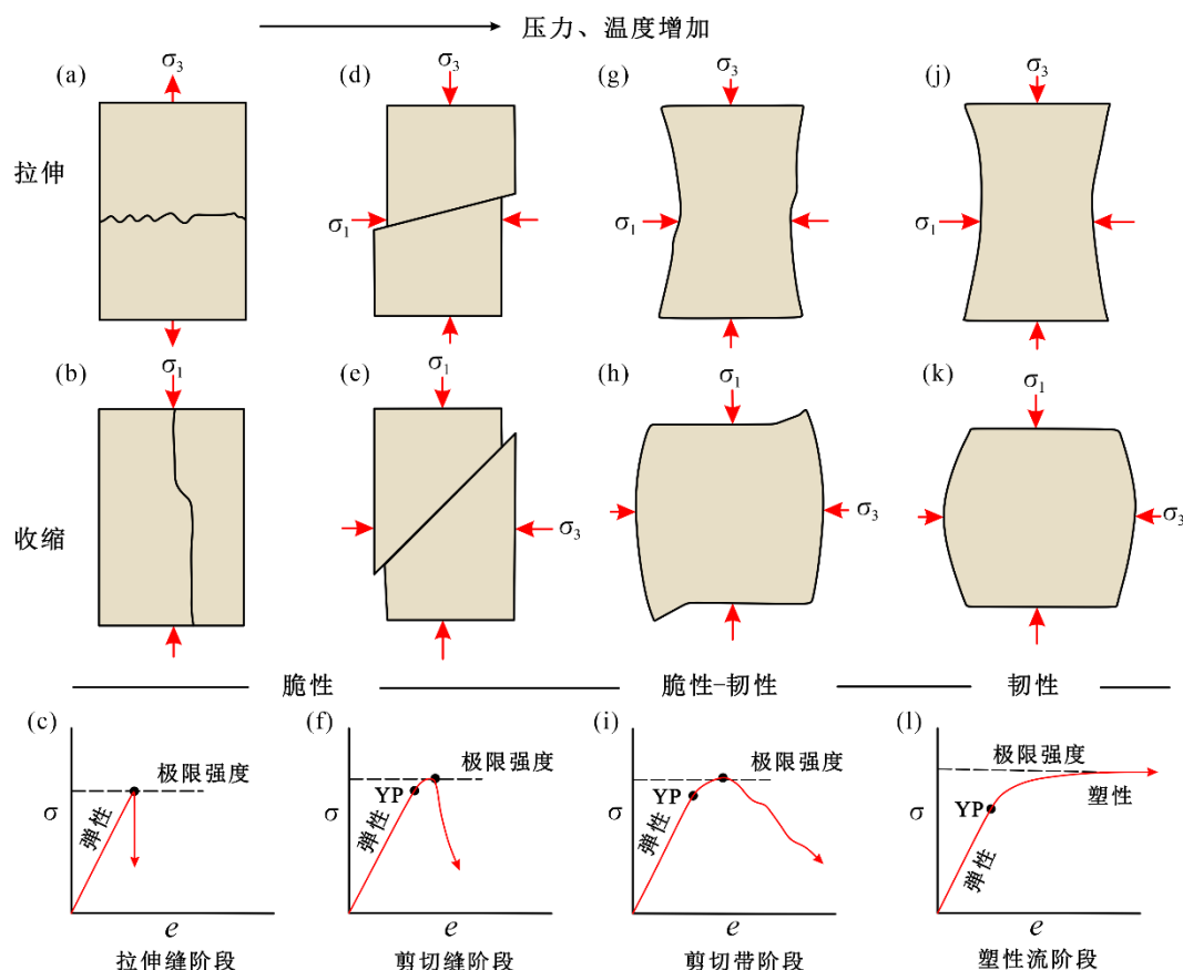
图 4 温度和围压对岩石力学性能的影响效应（据 Fossen，2016）
