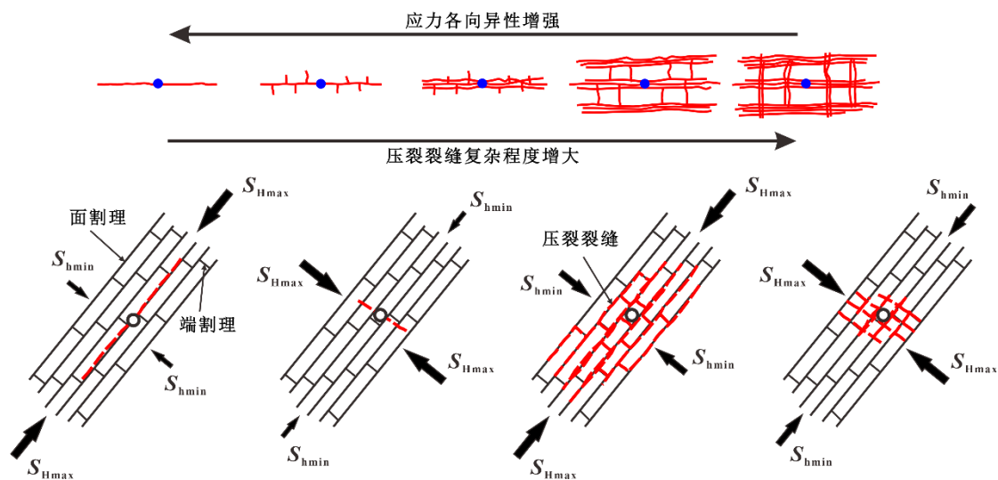
图2 受地应力非均质性和天然裂缝影响下的压裂裂缝扩展样式图 (据 Rajabi et al., 2017)
