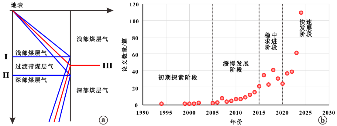
图1 深浅煤层气划分示意图 (a; 据 Qin et al., 2018) 与中国深部煤层气发展阶段图 (b; 据鞠玮等，2025) 图中：I 为吸附气含量临界深度小于地应力机制转换深度，此时地应力机制转换深度为深浅煤层气界线；II 为吸附气含量临界深度大于地应力机制转换深度，此时吸附气含量临界深度为深浅煤层气界线；III 为吸附气含量临界深度与地应力机制转换深度相等，此时任一深度为深浅煤层气界线。
