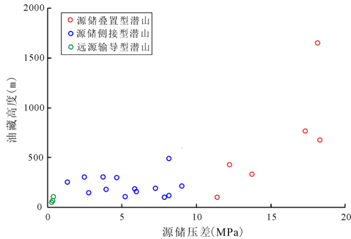
图 11 源-储压差与油藏高度的关系图
