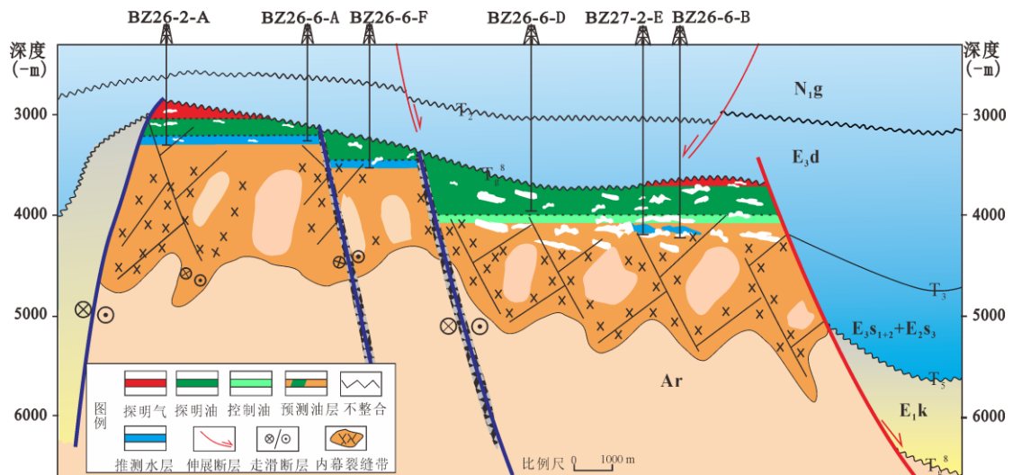
图 9 渤中 26-6 潜山成藏模式图
