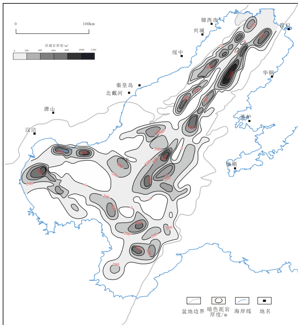
图 2.渤海海域沙三段烃源岩厚度分布图
