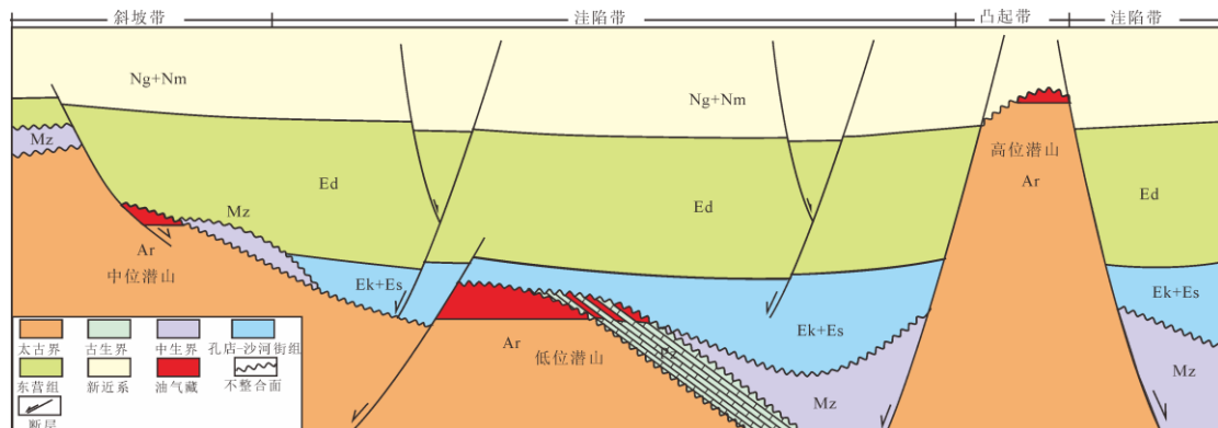
图 6 渤海海域中南部源-储配置关系与潜山类型划分
