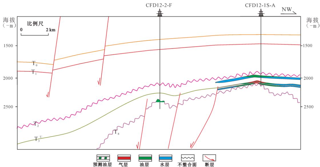
图 10 曹妃甸 12-2 潜山成藏模式图
