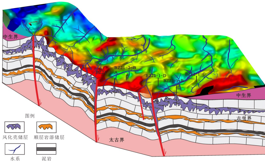
图 4 渤海海域古生界潜山成储模式图
