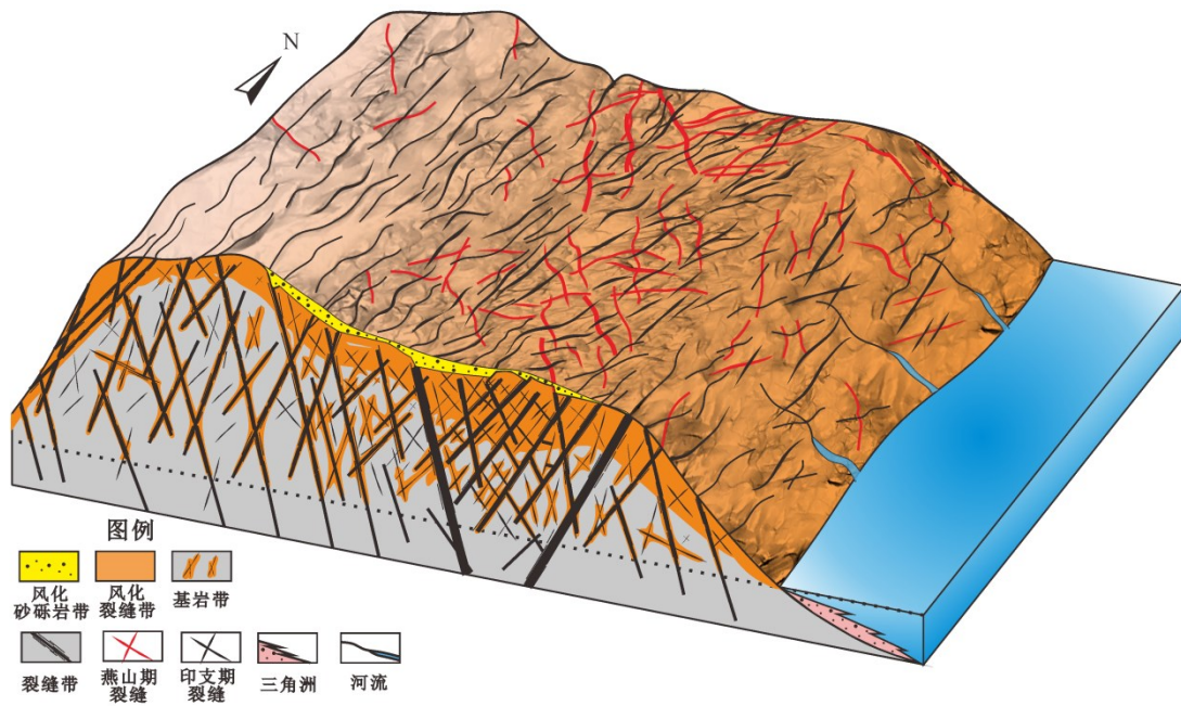
图 3 渤海海域太古界潜山成储模式图
