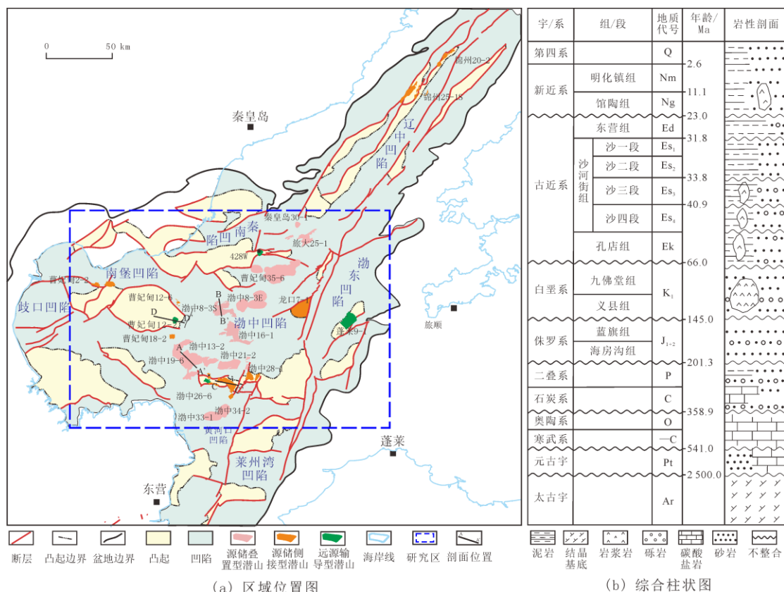
图 1 渤海海域潜山勘探区域图 (a) 和地层综合柱状图 (b)
