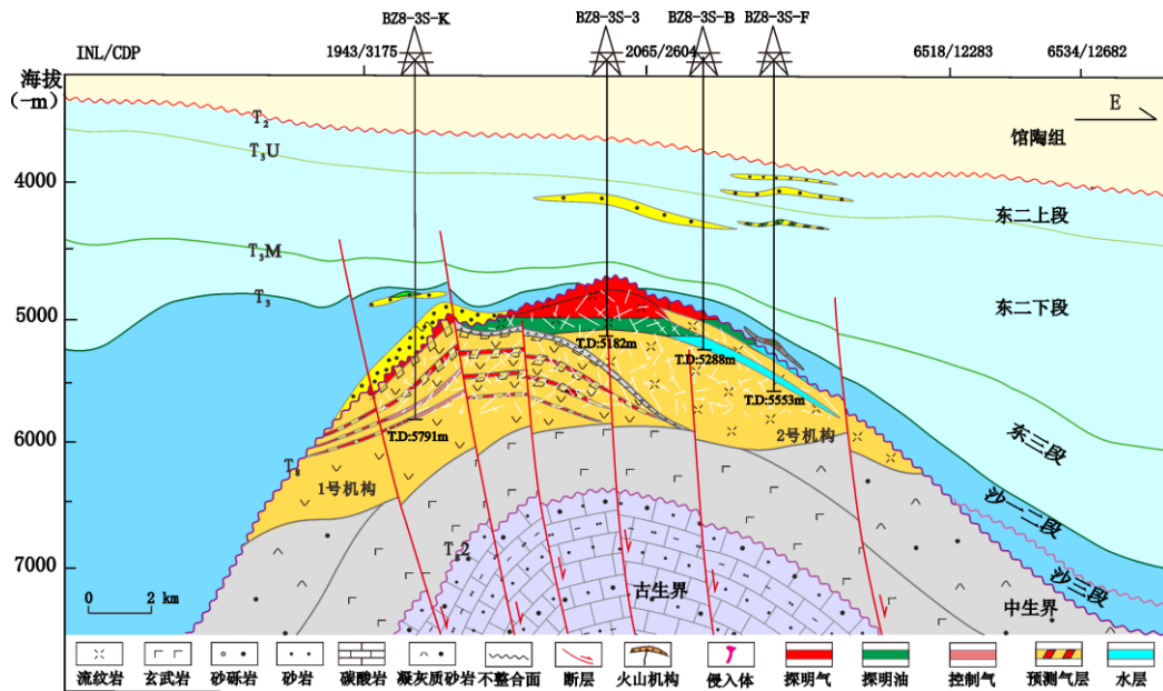
图 8 渤中 8-3S 低位潜山成藏模式图
