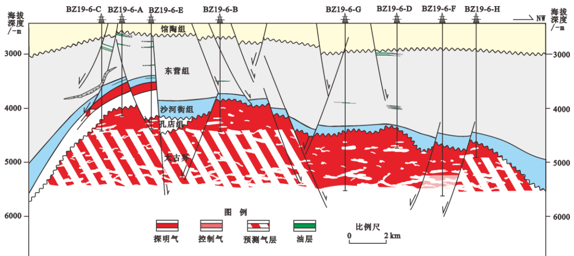
图 7 渤中 19-6 低位潜山成藏模式图
