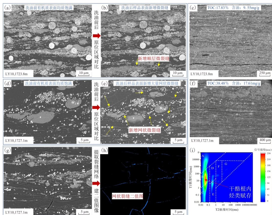
(a) 洗油前干酪根表面均质饱满, LY10 井 1723.8m; (b) 洗油后新增顺层微裂缝, LY10 井 1723.8m; (c) “无机纹层”包裹“有机纹层”叠置互层, LY10 井 1723.8m; (d) 洗油前干酪根表面均质饱满, LY10 井 1727.1m; (e) 洗油后新增网状微裂缝, LY10 井 1727.1m; (f) “有机纹层”包裹“无机纹层”叠置互层, LY10 井 1727.1m; (g) 干酪根内网状微裂缝形貌图; (h) 干酪根内网状微裂缝二值化图像; (i) 页岩型页岩油储层样品核磁共振 T_1 - T_2 信号图
