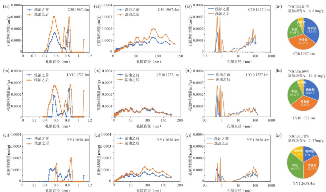
(a 1 , b 1 , c 1 ) 洗油前后微孔孔隙体积分布曲线对比, 基于洗油前后低温 CO 2 吸附实验; (a 2 , b 2 , c 2 ) 洗油前后介孔-宏孔孔隙体积分布曲线对比, 基于洗油前后低温 N 2 吸附实验; (a 3 , b 3 , c 3 ) 洗油前后联孔孔隙体积分布曲线对比; (a 4 , b 4 , c 4 ) TOC、氯仿沥青 A 与烃类族组成特征
