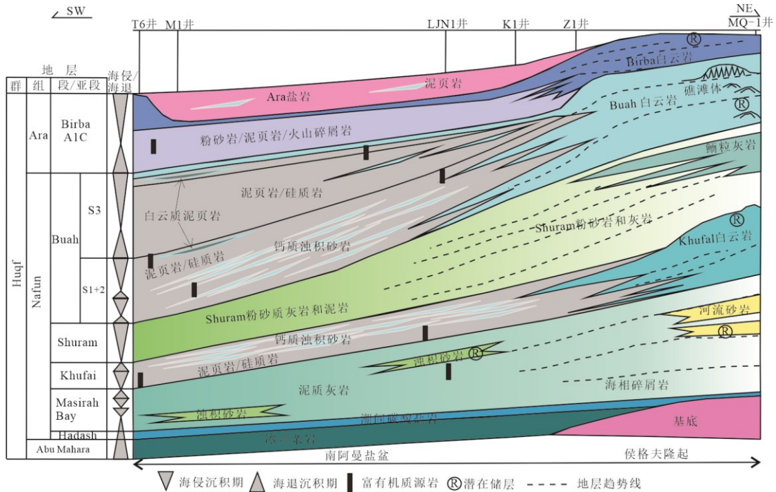
图 3 阿曼盆地南部前寒武系-下寒武统海侵-海退旋回与地层沉积（改自 Gómez-Pérez et al. , 2024）
