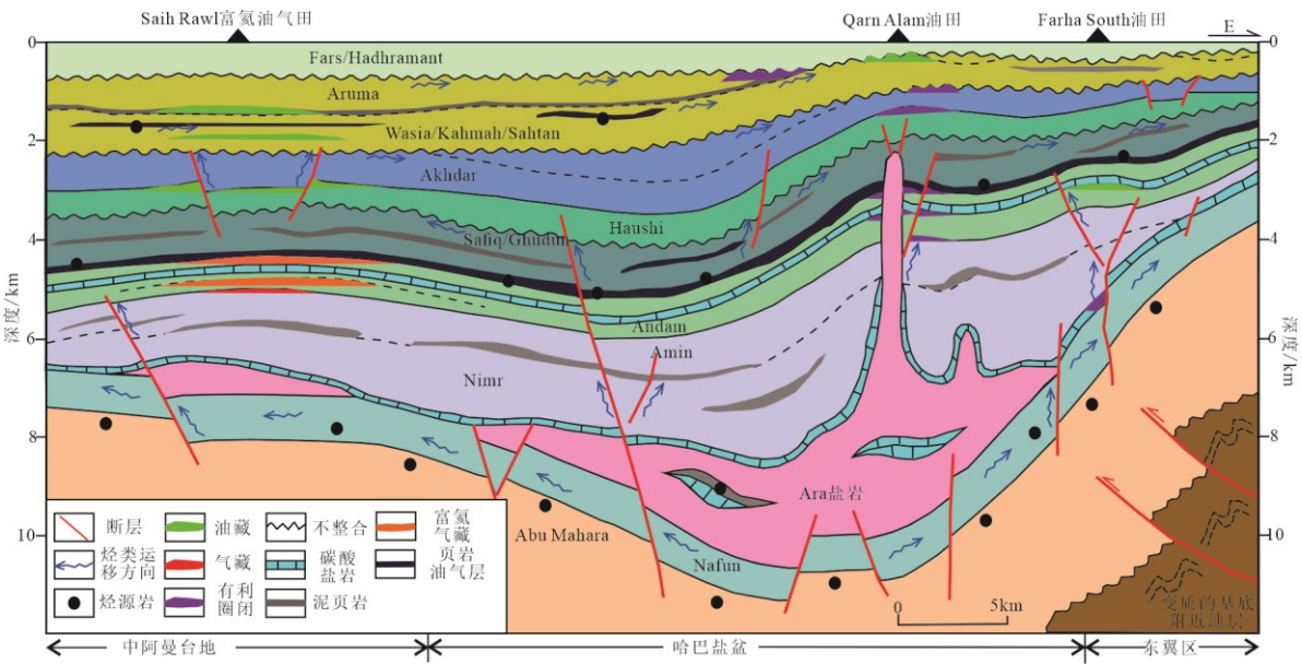
图 8 阿曼盆地哈巴盐盆周缘油气运移模式图（改自 Droste, 1997）(剖面位置见图 1BB’) Fig.8 Hydrocarbon migration pattern map around the Ghaba salt basin in Oman Basin
