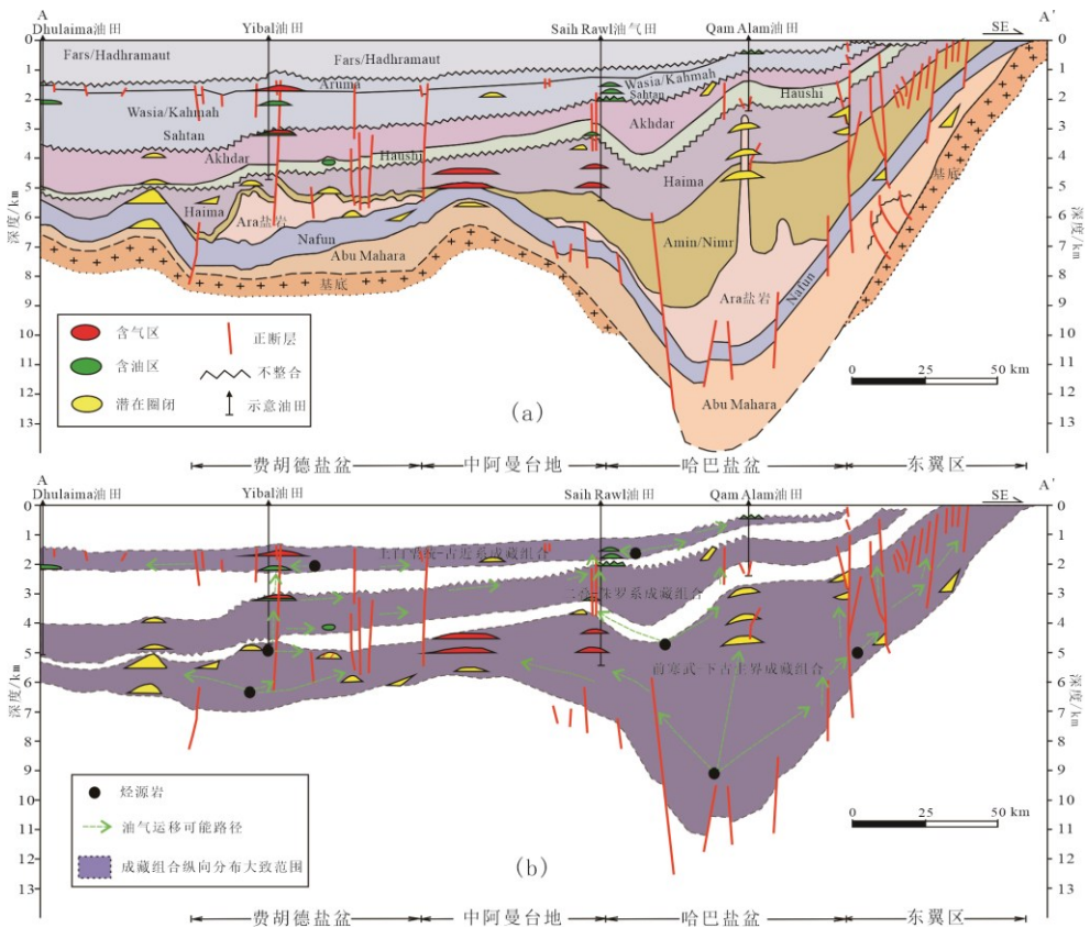
图 5 阿曼盆地北部地质剖面（a）和成藏组合划分（b）（a 改自 Ai-Husseini, 1997，剖面位置见图 1b） Fig.5 Geological profile of the northern Oman Basin (a) and division of petroleum systems (b)
