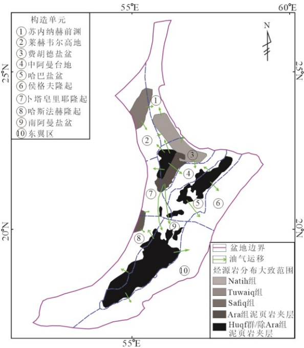
图 6 阿曼盆地烃源岩分布与油气运移示意图（烃源岩分布据 Terken et al. , 2001）
