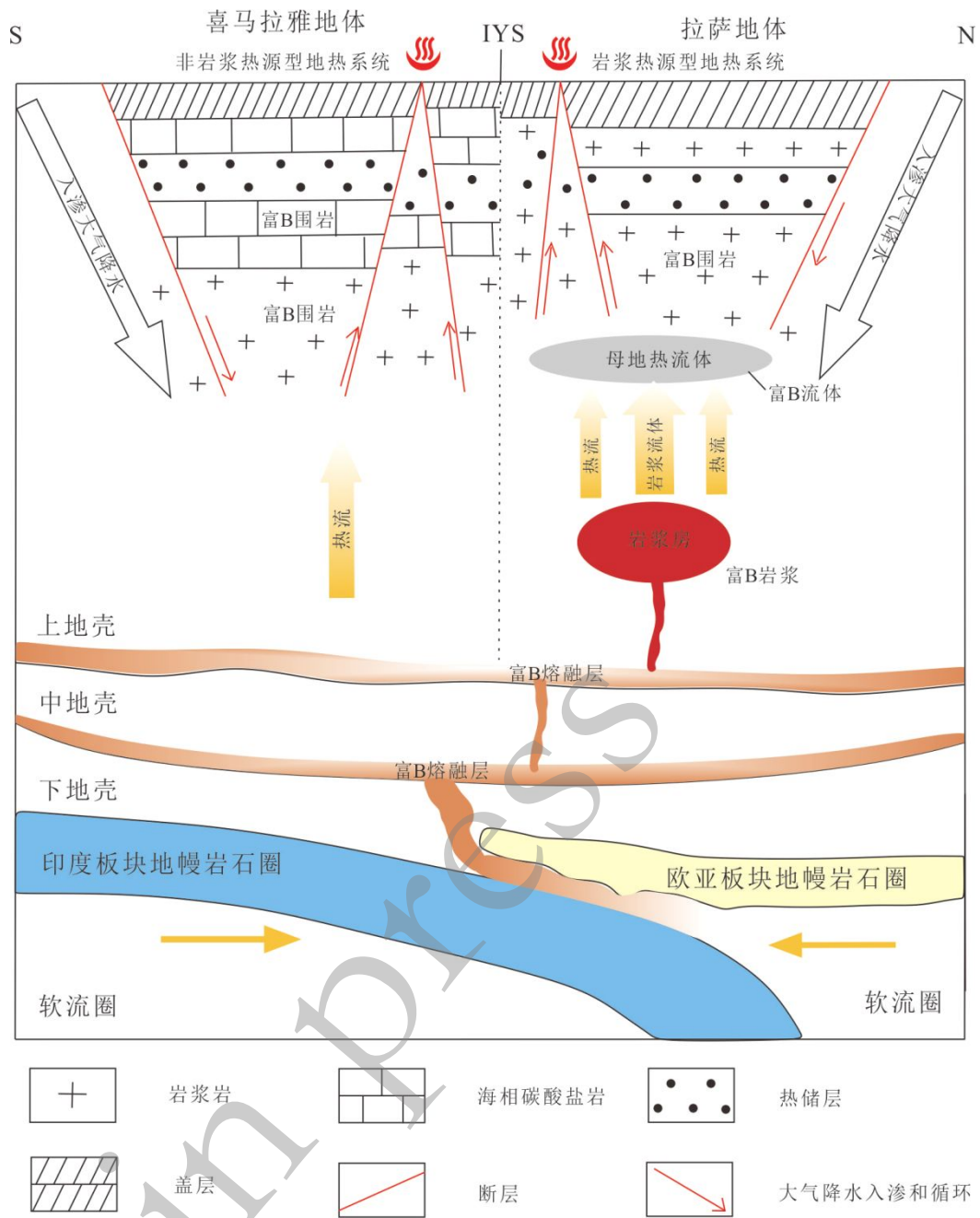
图 2 西藏地热水中硼富集机制图 (改编自 Liu et al., 2019)
