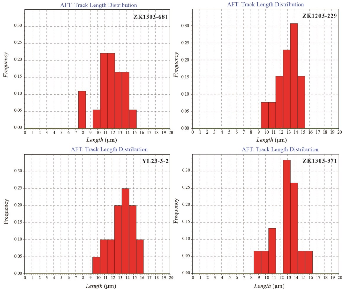
图 7 围陷径迹长度分布图
