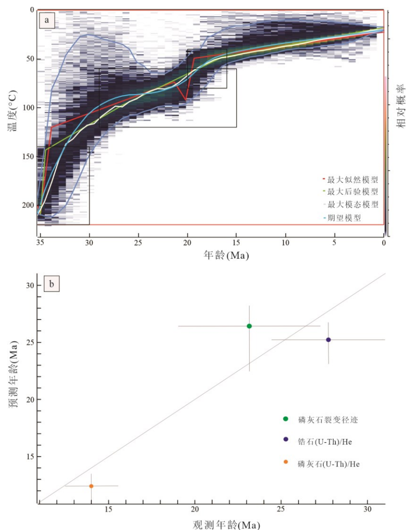
图 10 玉龙矿床热史反演模拟结果 (a) 及年龄预测 (b)
