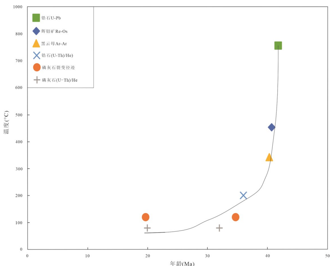
图 12 玉龙矿床热历史演化图
