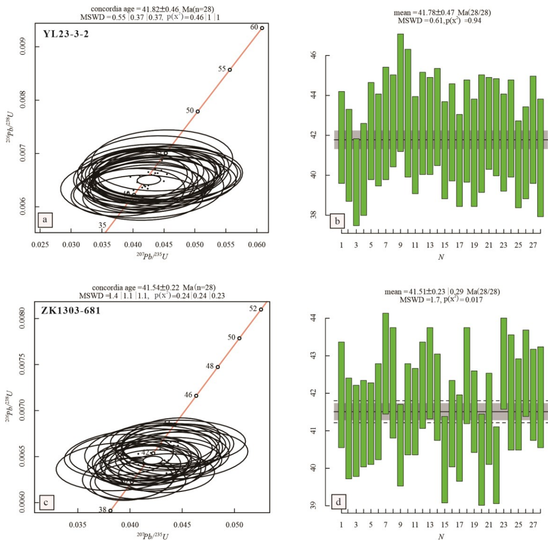
图 6 锆石 U-Pb 谐和年龄及加权平均年龄图
