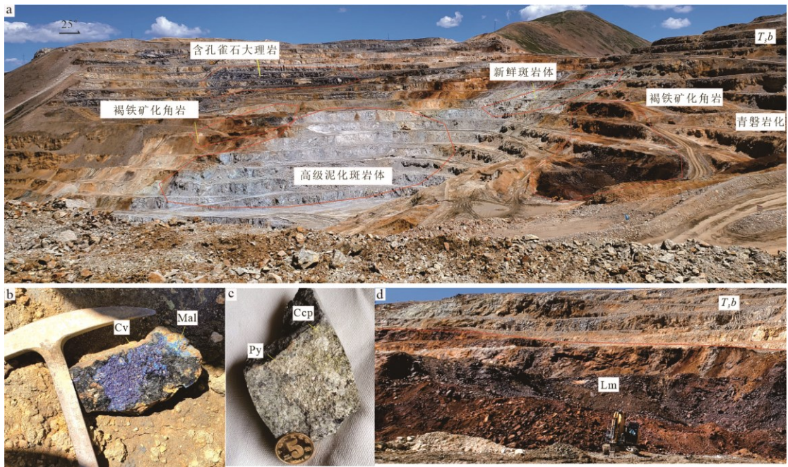
图 3 玉龙矿床露头采坑和代表性矿石
