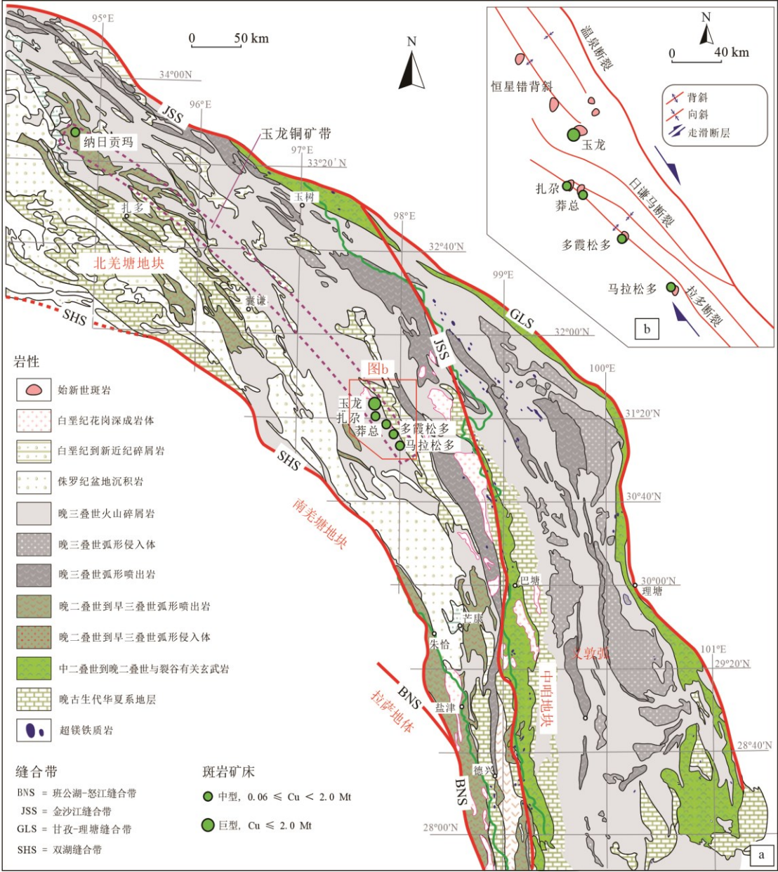
图 1 三江北段地质图 (a)玉龙斑岩铜矿带南段构造和斑岩分布简图(b) (据 Yang and Cooke, 2019 修改)
