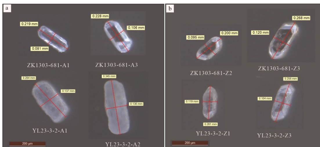
图 9 用于(U-Th)/He 测试的磷灰石颗粒尺寸照片 (a) 用于(U-Th)/He 测试的锆石颗粒尺寸照片 (b)
