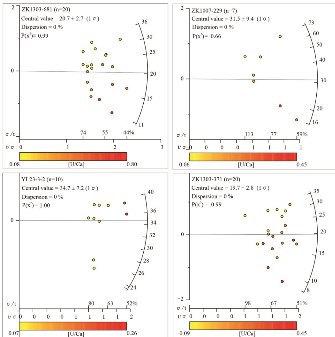
图 8 二长花岗斑岩磷灰石裂变径迹年龄雷达图
