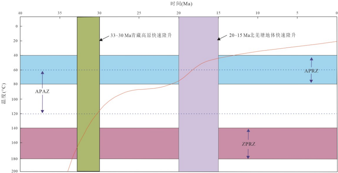
图 13 玉龙矿床热历史模拟最佳曲线与区域构造事件图
