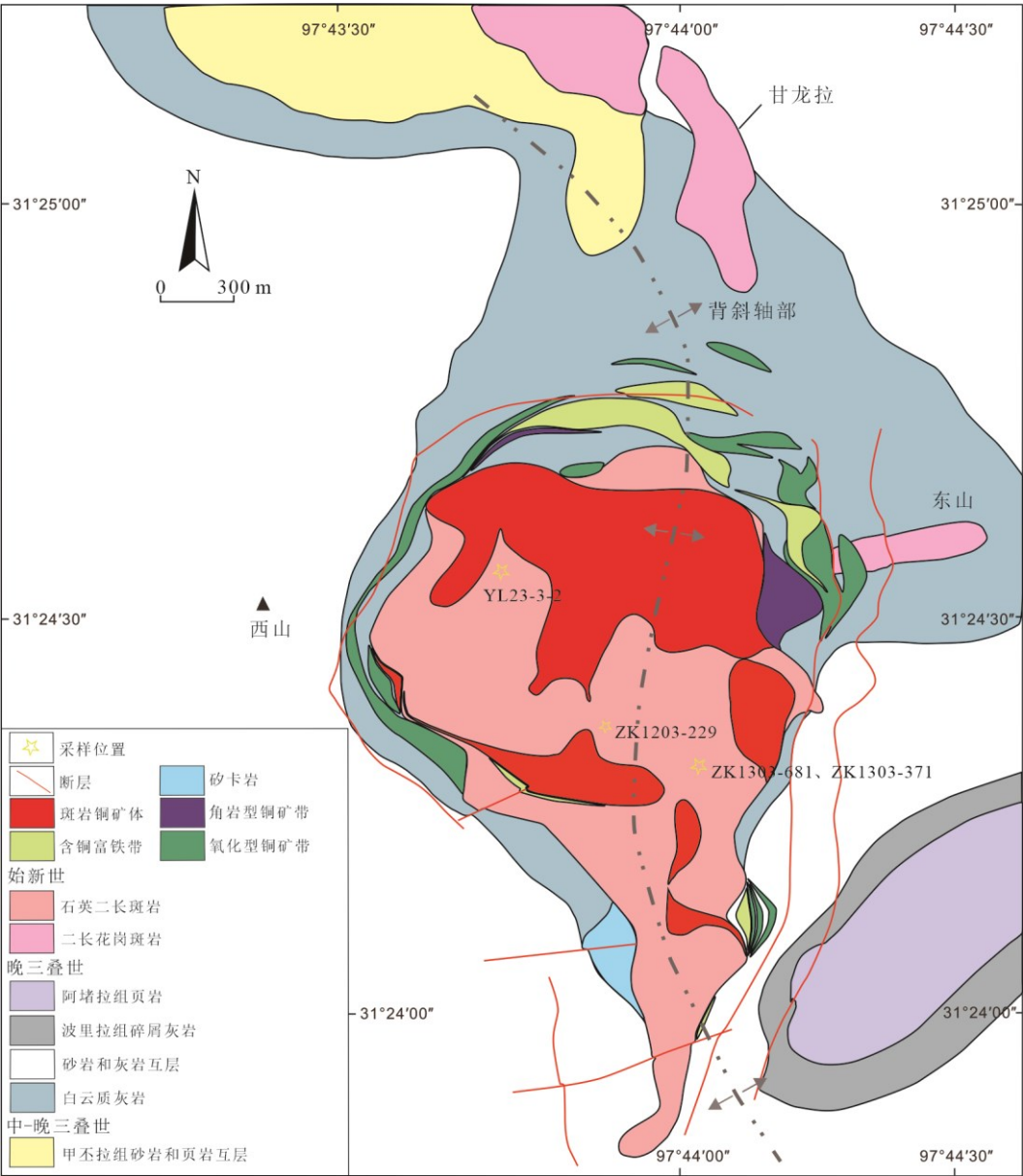
图 2 玉龙矿区地质图（据 Chen et al., 2021 修改）
