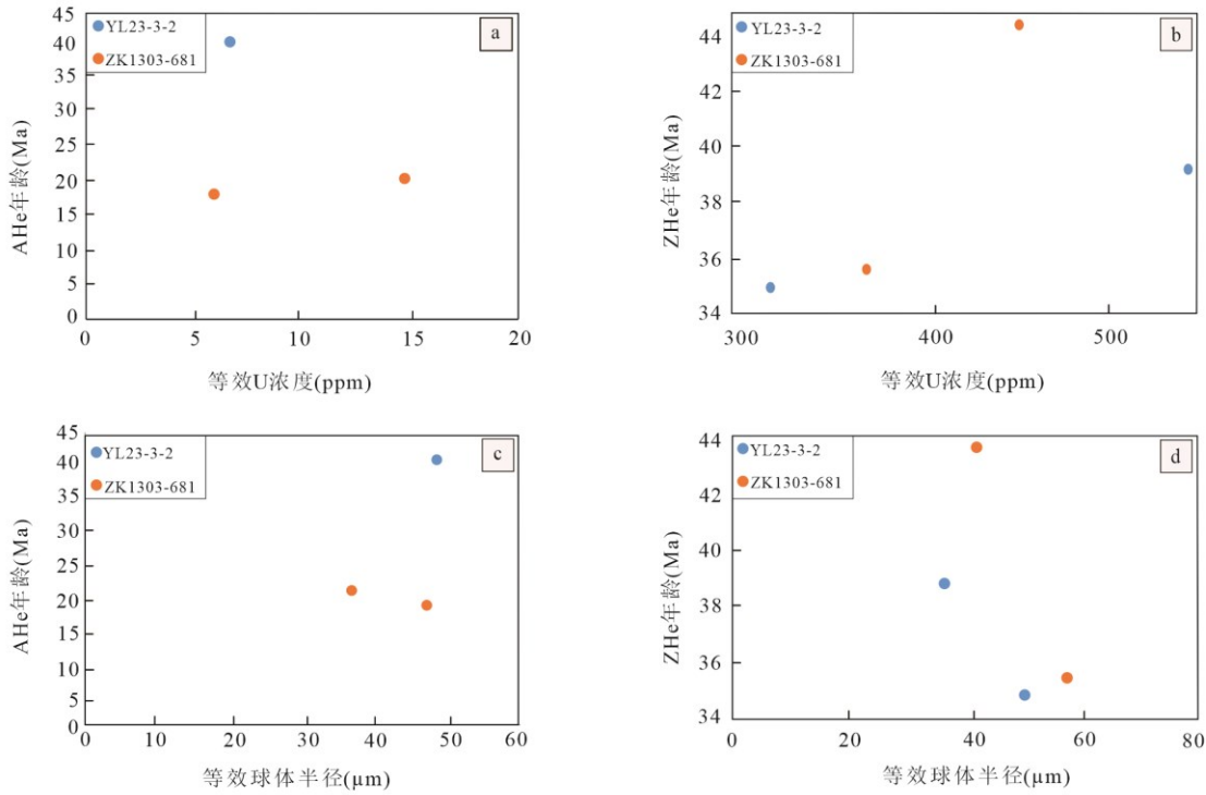
图 11 (U-Th)/He 年龄-等效 U 浓度图（a, b）(U-Th)/He 年龄-等效球体半径图（c, d）
