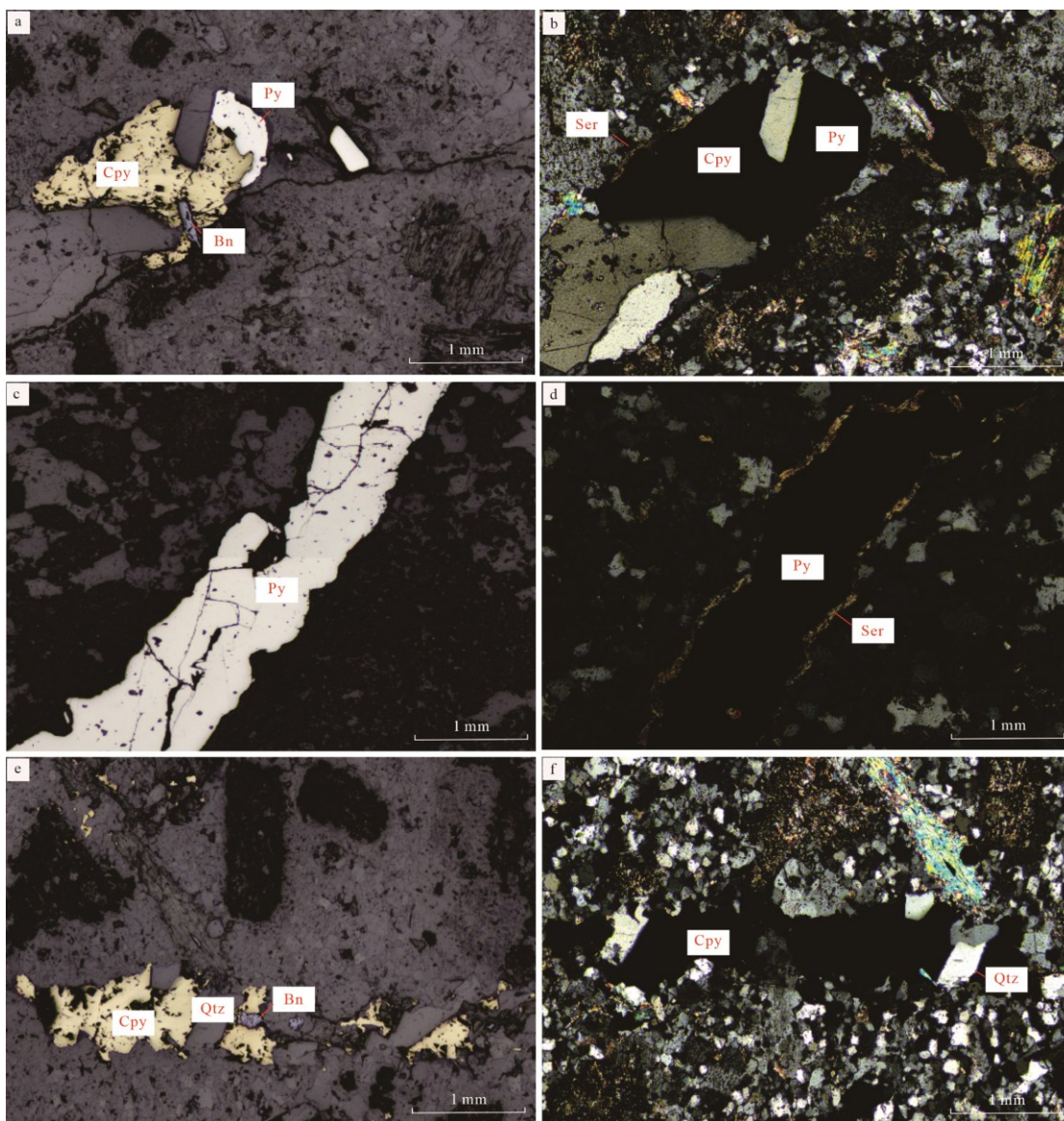
图 4 典型原生矿石镜下照片
