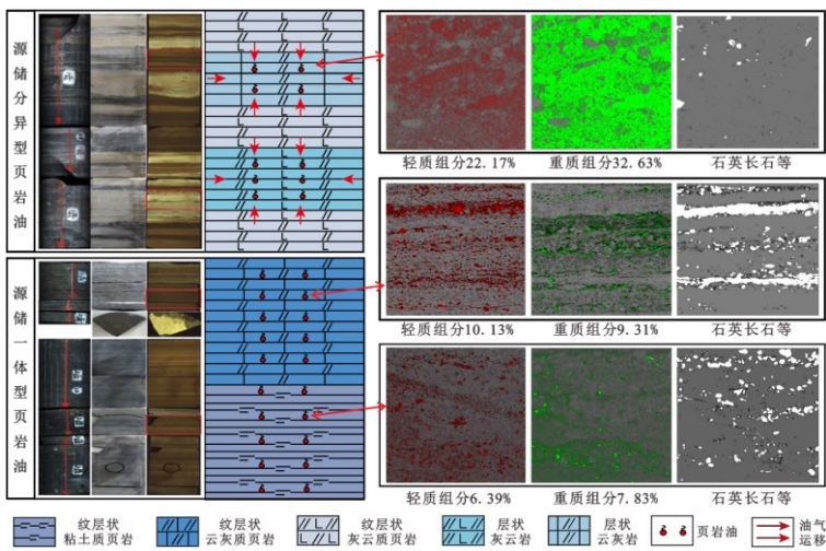
图 11 下干柴沟组上段源储组合类型及其含油性示意图，右图为激光共聚焦显微镜照片，揭示了页岩油差异分布特征，修改自李国欣，2023c
