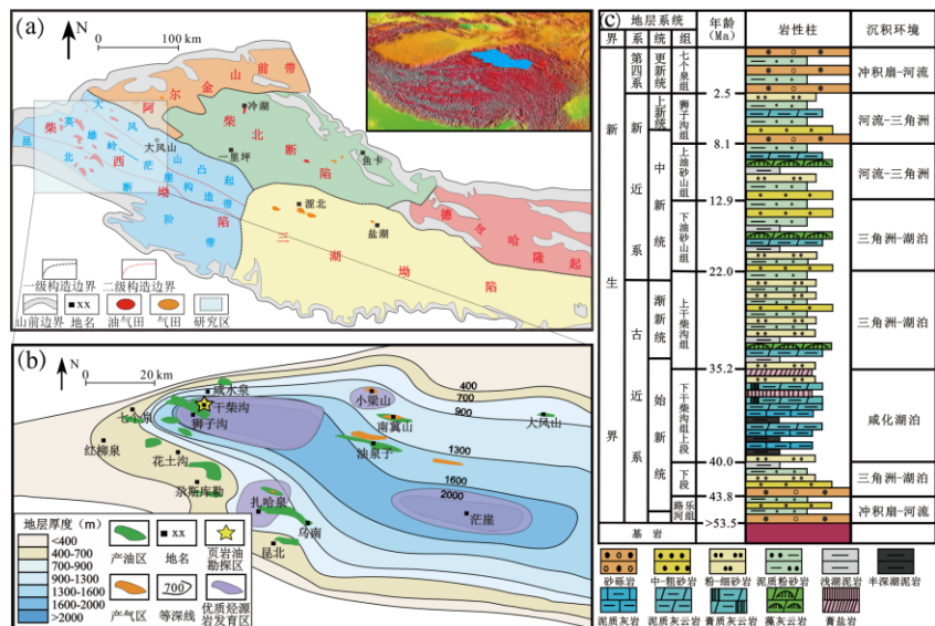
图 1 柴达木盆地构造单元与地层分布特征图，修改自青海油田内部资料（a）柴达木盆地构造单元划分及油气田分布；（b）柴西坳陷下干柴沟组上段地层厚度及油气分布；（c）柴西坳陷地层综合柱状图
