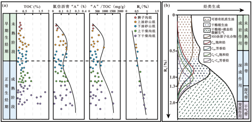
图 9 柴西坳陷咸化湖相烃源岩生烃模式图，(a) 咸 8 井自然生烃演化剖面，修改自彭德华，2004；(b) 未熟-成熟二段式生烃模式图，修改自李国欣等，2023b
