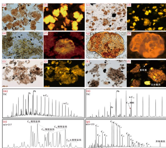
图5 下干柴沟组上段沉积期间的生物种群特征，来自有机岩石学和生物标志化合物的指示，显微照片拍摄于透射光和蓝光激发的荧光条件下。（a-d）葡萄藻，据 Zhang et al., 2023；（e-f）疑源类，据邢蓝田，2022；（g-h）双气囊花粉，据 Zhang et al., 2023；（i-l）柴908井宏体藻类；（m）跃灰10X井烃源岩饱和烃总离子流图，据 Zhang et al., 2023；（n）：跃灰103井烃源岩饱和烃总离子流图（部分），高丰度的高支链类异戊二烯炔（C 25 HBI）指示了硅藻的贡献，据张永东等，2011；（o）柴906井烃源岩饱和烃甾烷类化合物谱图，据郝万鑫等，2023；（p）柴10井烃源岩芳烃类化合物谱图，高丰度芳基类异戊二烯炔和异海棉烷的检出指示了绿、紫硫细菌对有机质的改造作用，据郝万鑫等，2023
