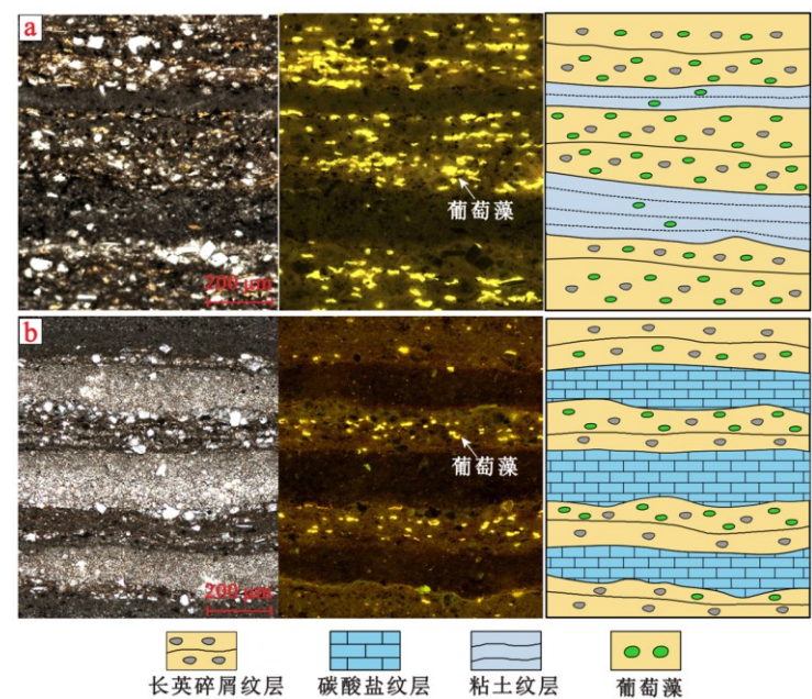
图 6 下干柴沟组上段纹层型页岩的岩石学特征与葡萄藻分布示意图，显微照片拍摄于反射光和蓝光激发的荧光条件下，修改自 Zhang et al., 2023
