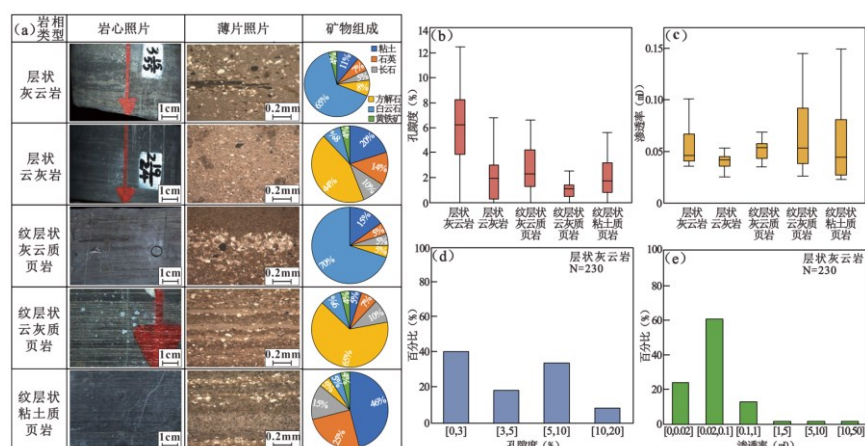
图 10 下干柴沟组上段不同岩相储层岩石学特征及物性特征差异示意图，物性评价参数为页岩柱塞样测定的氦气孔隙度和空气渗透率，修改自邢浩婷等，2024
