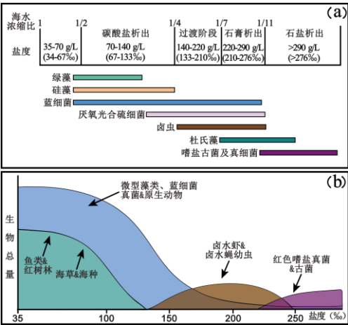
图 2 现代高盐度水体 (海洋、咸水湖泊) 盐度与生物发育特征的协同变化规律示意图。(a) 典型微生物的盐度耐受范围，海水浓缩比为盆地的流入量与盆地内包括蒸发和退潮在内的流出量之比，g/L 与 psu 盐度的换算假定海水密度为 1.05 g/cm 3 ，修改自 Barbe et al. , 1990; (b) 现代海洋不同盐度范围水体对应的生物种类与总量，修改自 Warren, 2011
