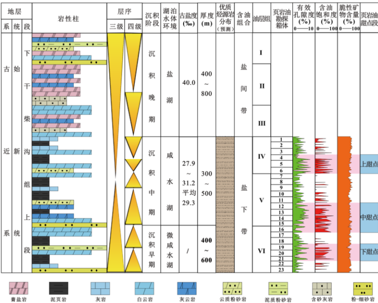
图 8 下干柴沟组上段沉积环境演变与页岩油甜点段分布示意图 (修改自 Wang et al., 2020)
