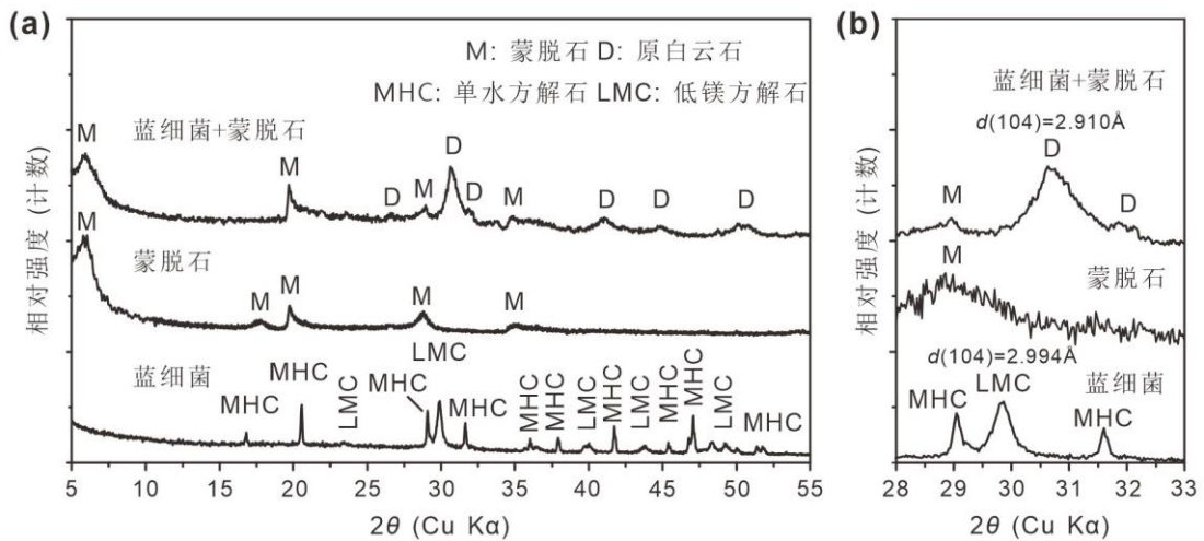
图1 有无蒙脱石条件下蓝细菌矿化产物的XRD图谱：（a）全谱图；（b）28-33° 2\theta 局部放大
