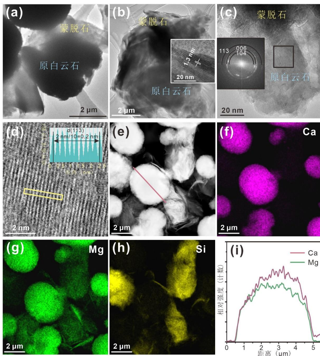
图6 黏土矿物存在条件下反应体系最终产物的TEM分析: (a-c) 蒙脱石-原白云石聚集体, 其中(b)和(c)的插图分别显示了蒙脱石的高分辨晶格条纹以及原白云石的电子衍射谱; (d) 原白云石(113)晶面的高分辨晶格条纹; (e-h) 蒙脱石-原白云石聚集体的元素分布图, 其中(f)、(g)和(h)分别对应Ca、Mg和Si的元素分布; (i) 沿(e)中实线扫描路径获得的原白云石颗粒中Ca和Mg元素的EDS线扫描分布
