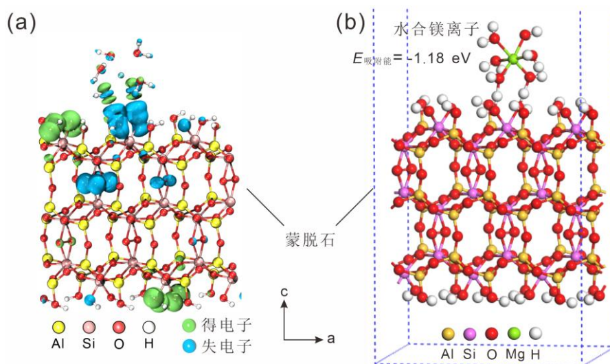
图7 DFT模拟蒙脱石水合镁离子的吸附过程：(a) 蒙脱石表面差分电荷图；(b) 羟基位点与水合镁离子的配位构型
