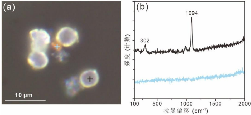
图2 蒙脱石存在条件下蓝细菌矿化产物形貌 (a) 及拉曼图谱 (b)
