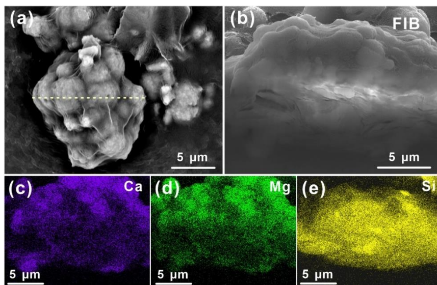
图5 蒙脱石条件下蓝细菌矿化反应体系产物的FIB-SEM-EDS图谱：(a) 蒙脱石-原白云石聚集体，其中虚线显示切割位置；
