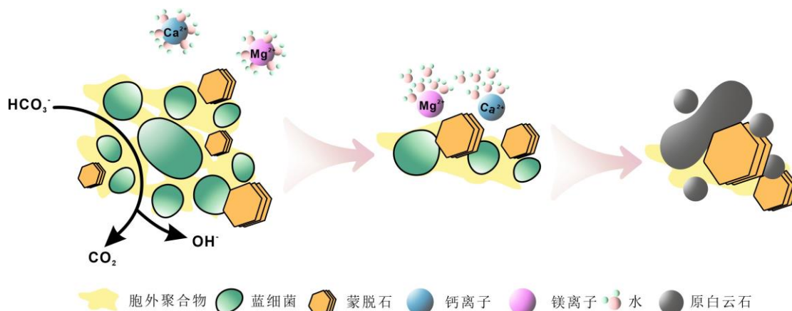
图8 蓝细菌-蒙脱石协同介导原白云石形成过程的示意图
