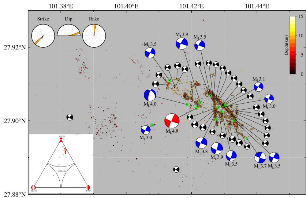
图 4 震源机制解、地震类型三角形图解及节面参数统计分布图
