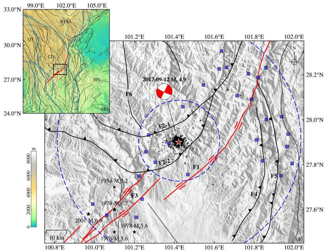
图 1 木里地震震源区构造分布图
