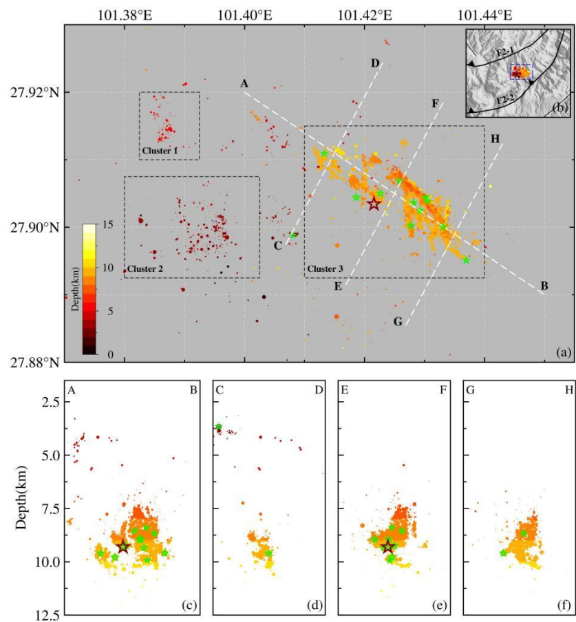
图 3 地震序列分布图
