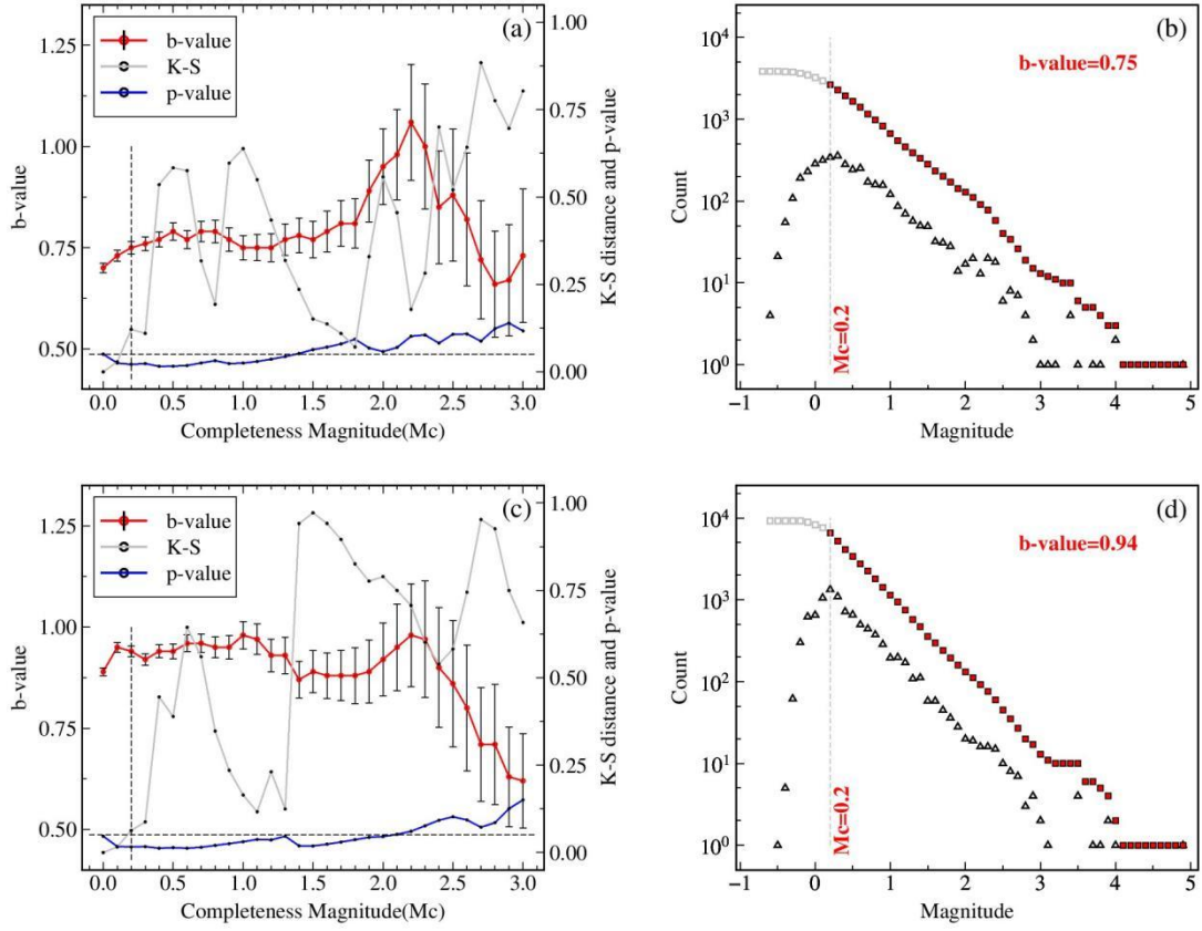
图 6 地震目录统计分析对比
