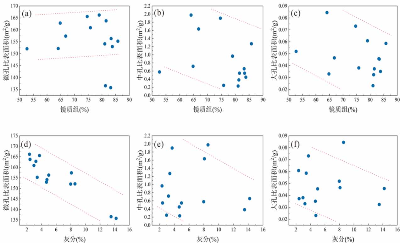
图 12 绥德 1H 井本溪组 8#煤镜质组、灰分与孔比表面积关系图
