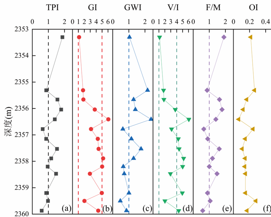
图 9 绥德 1H 井本溪组 8#煤储层煤相参数分析图
