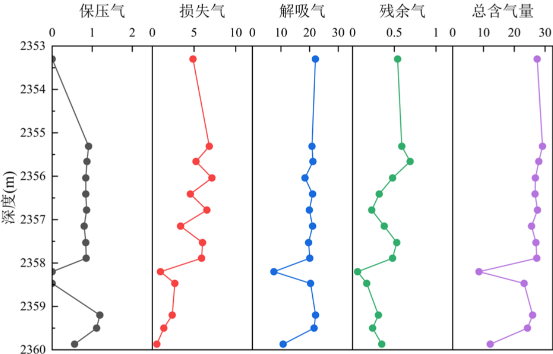
图 7 绥德 1H 井本溪组 8#煤储层含气量随深度变化图
