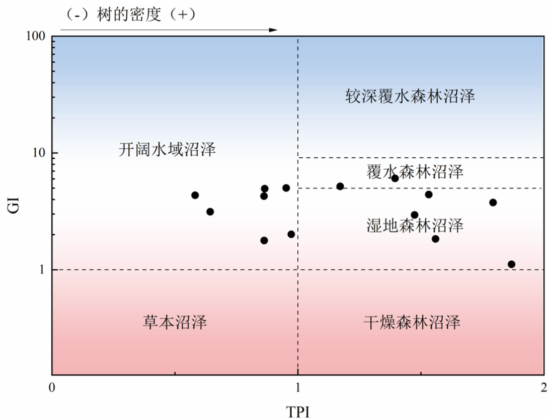
图 8 绥德 1H 井本溪组 8#煤储层 TPI-GI 煤相图
