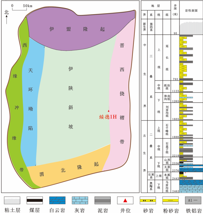
图 1 绥德 1H 井区域构造及地层柱状图
