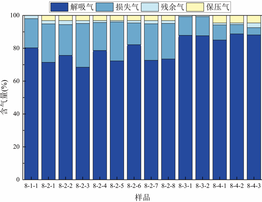
图 13 绥德 1H 井本溪组 8#煤含气量分布图
