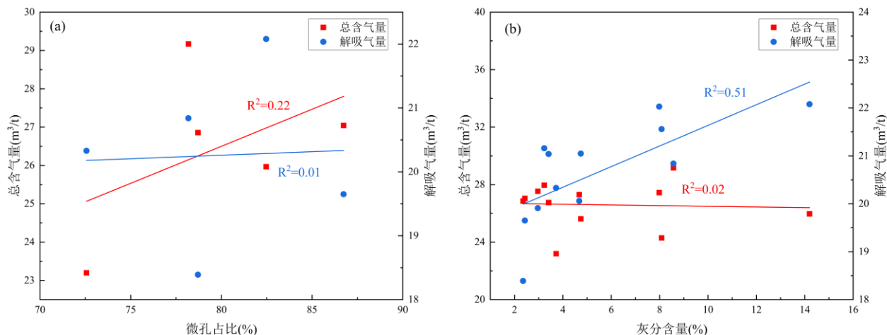
图 14 绥德 1H 井本溪组 8#煤微孔占比和灰分含量与总含气量和解吸气量关系图
