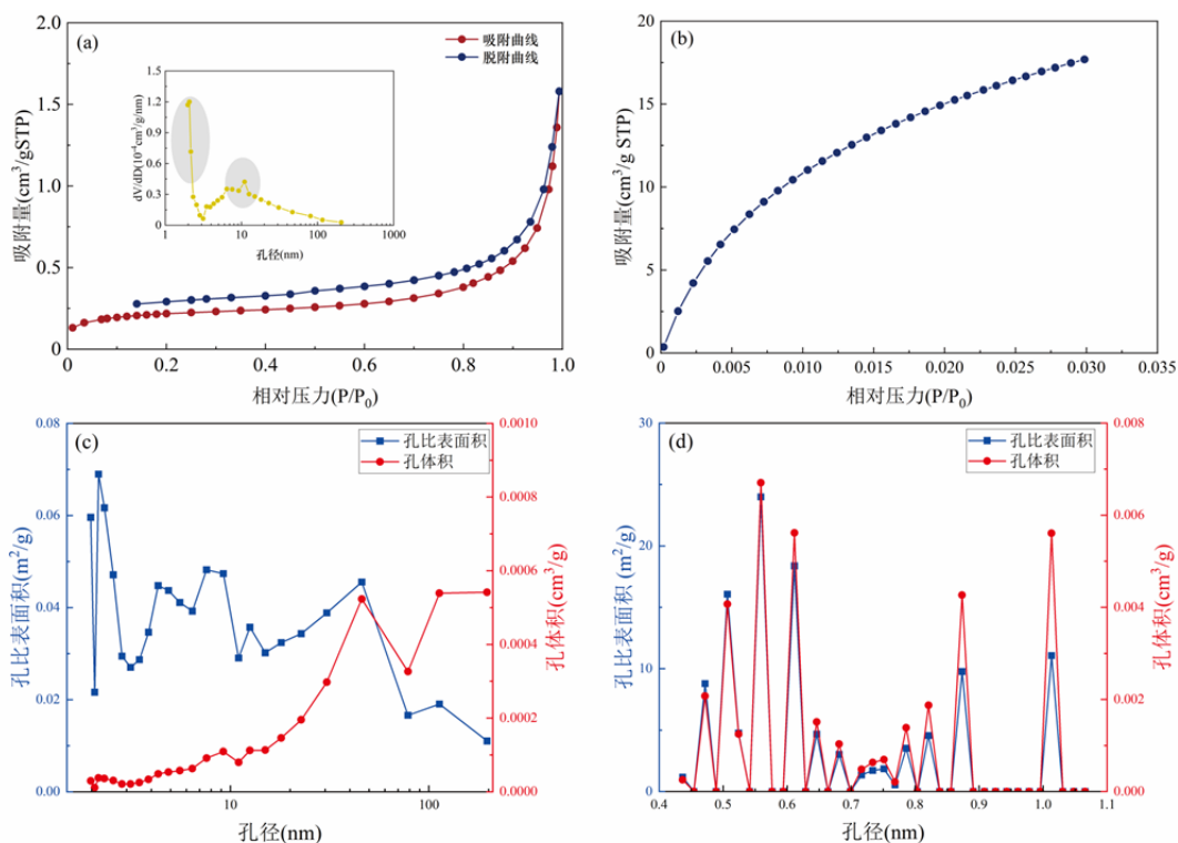
图 6 绥德 1H 井本溪组 8#煤岩储层孔隙特征分析图
