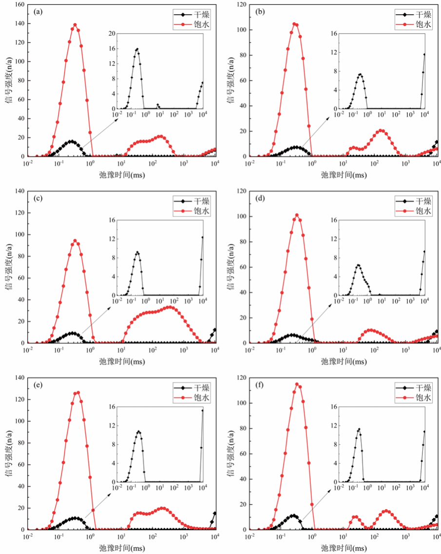
图 4 绥德 1H 井本溪组 8#煤岩储层核磁共振 T 2 谱图
