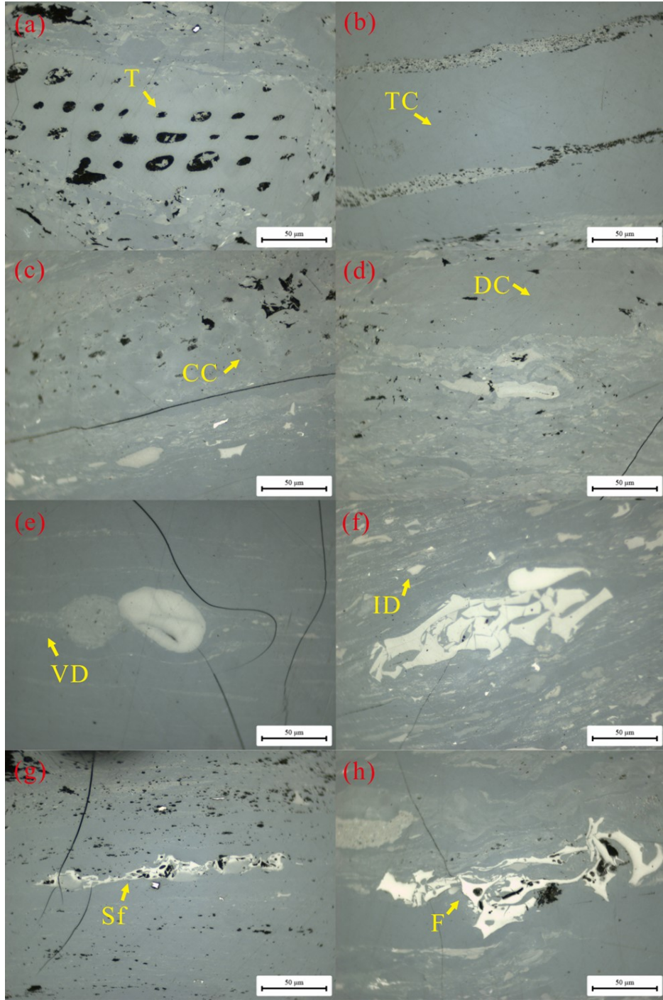
图3 绥德 1H 井本溪组 8#煤岩储层显微组分特征
