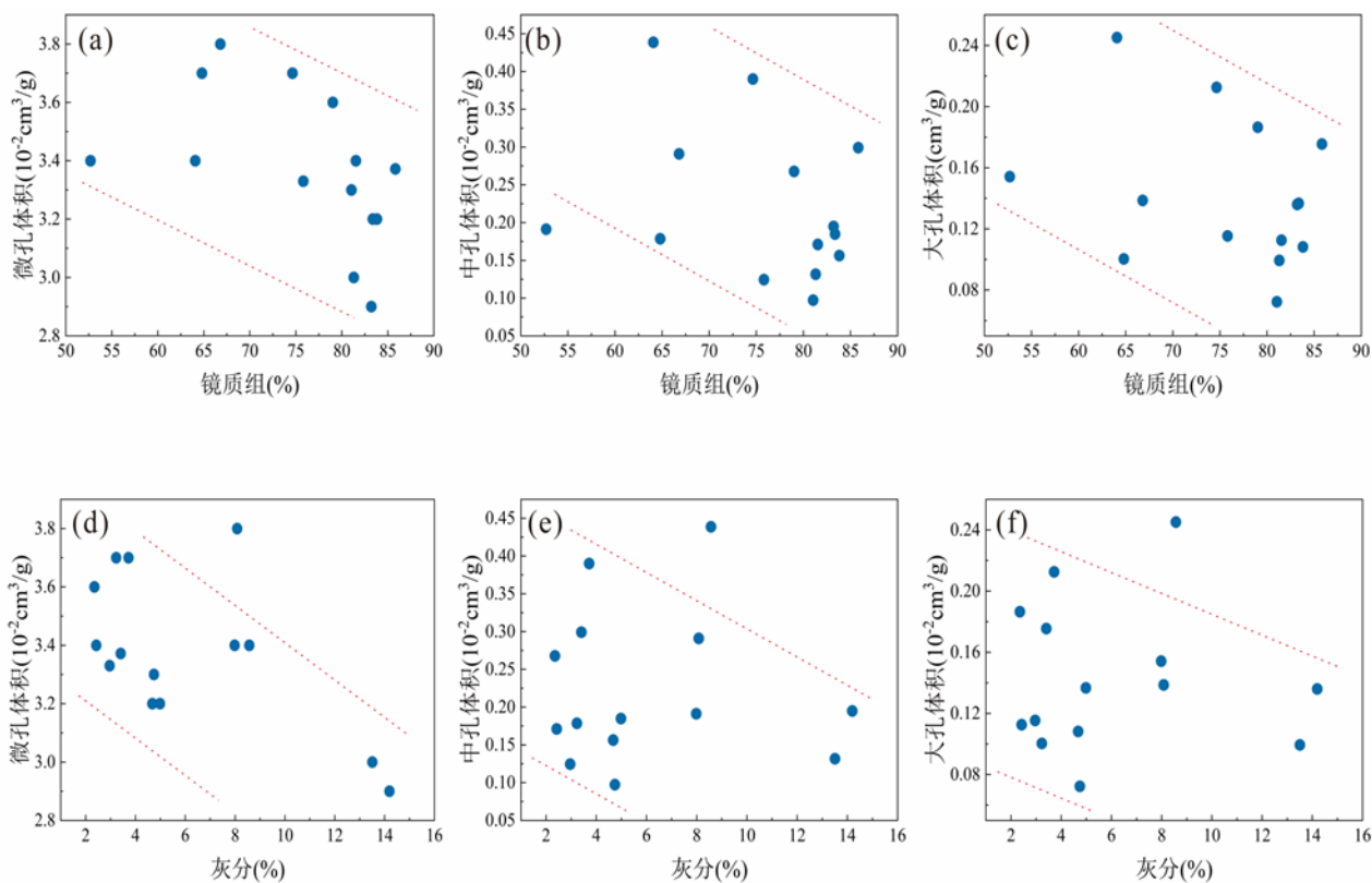
图 11 绥德 1H 井本溪组 8#煤镜质组、灰分与孔体积关系图
