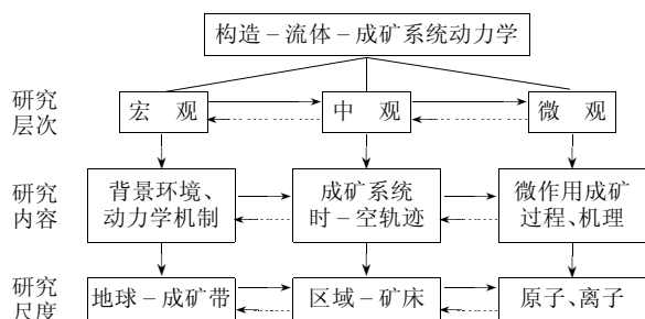
图 2 构造-流体-成矿系统及其动力学层次-整体性
