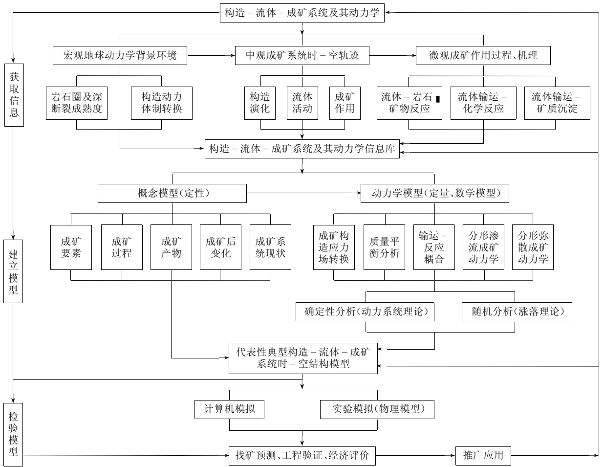
图 3 构造-流体-成矿系统及其动力学方法体系
