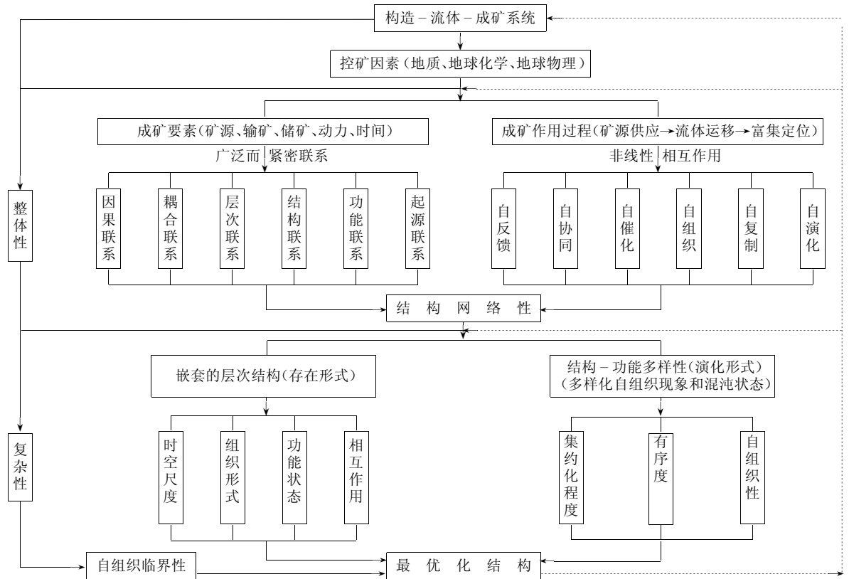
图 1 构造-流体-成矿系统理论格架
