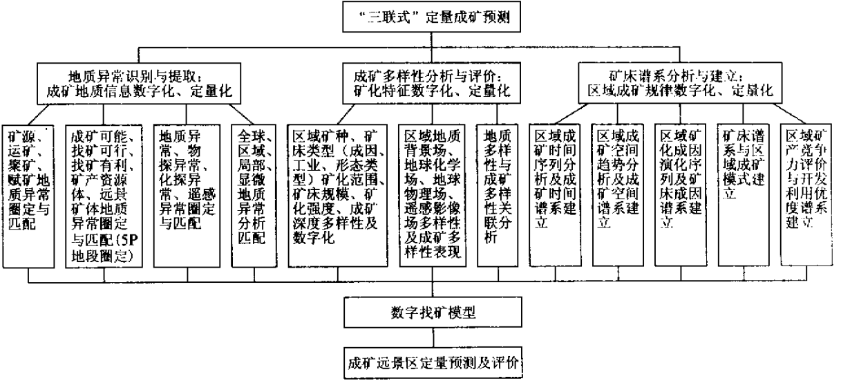
图 1 “三联式”定量成矿预测模型
