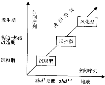
图2 不同成因类型重晶石矿成矿谱系
