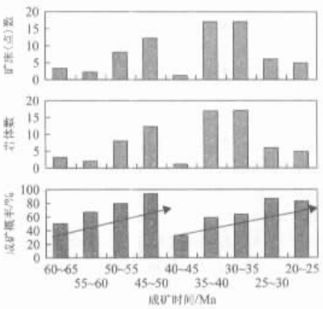
图3 滇西北富碱斑岩综合成矿时间谱系
