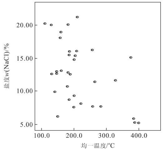
图 3 会泽铅锌矿床气液包裹体盐度-均一温度
