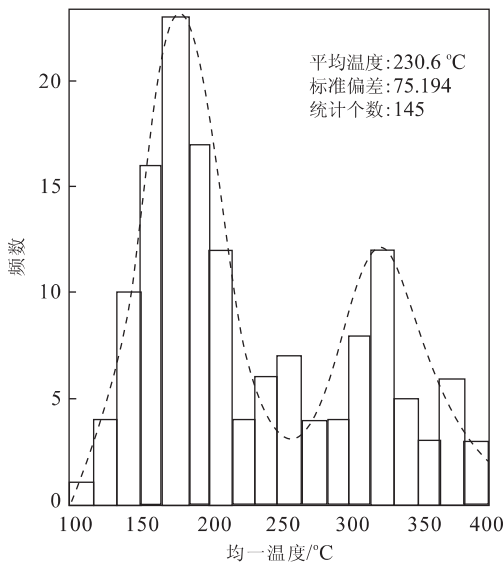
图 2 会泽铅锌矿床矿物流体包裹体均一温度分布
