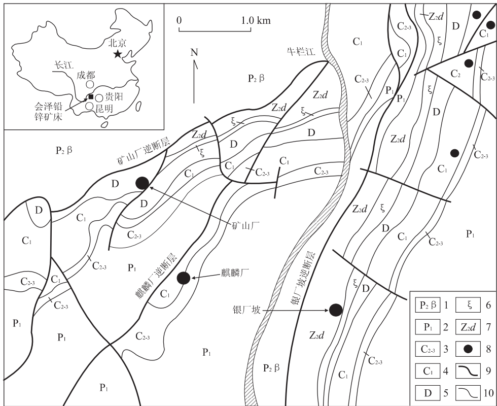
图 1 会泽铅锌矿床矿区地质图
