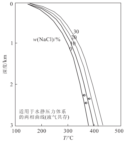
图 4 会泽铅锌矿床成矿深度 (据 Hass, 1971, 1976)
