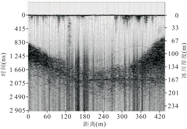
图 3 黑沟 8 号冰川 C1-C2 测线雷达图像 Fig. 3 Radar image along the sounding transect C1-C2 on Heigou glacier No. 8
