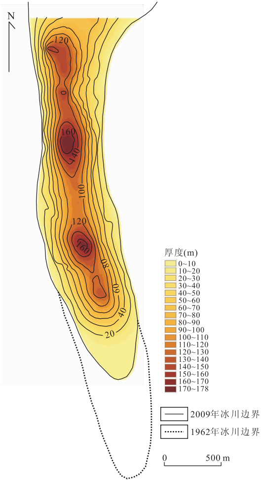
图 4 基于普通克里格法的黑沟 8 号冰川冰舌厚度分布及 1962—2009 年冰川末端变化
