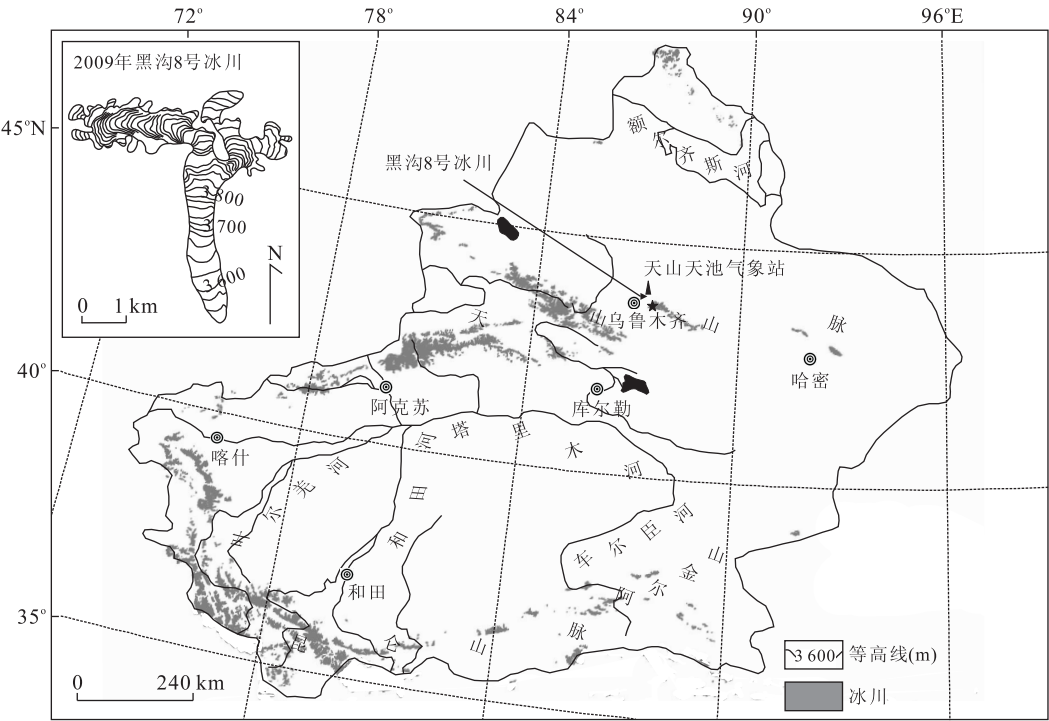
图 1 黑沟 8 号冰川位置 Fig. 1 Location map of Heigou glacier No. 8
