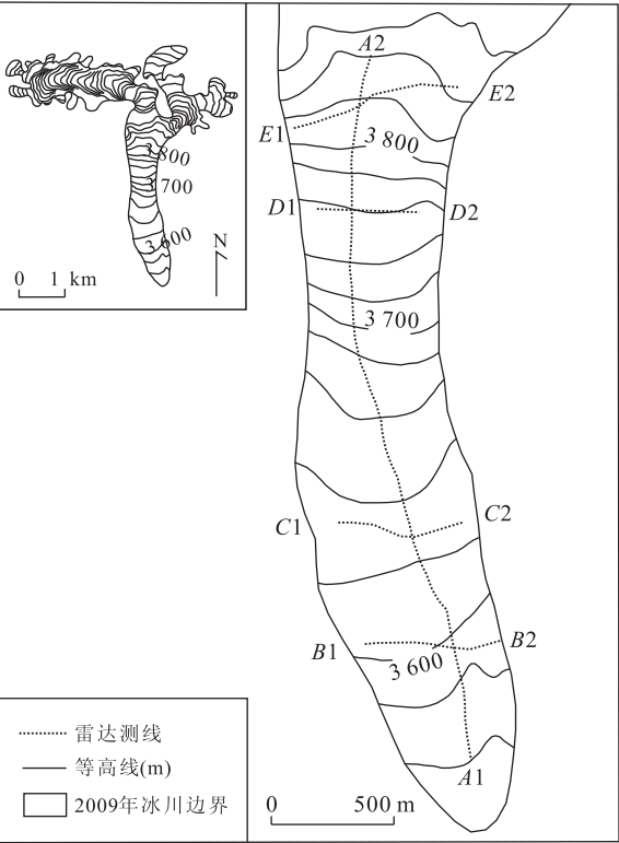
图 2 黑沟 8 号冰川雷达测厚路线分布 Fig. 2 GPR measuring lines of Heigou glacier No. 8
