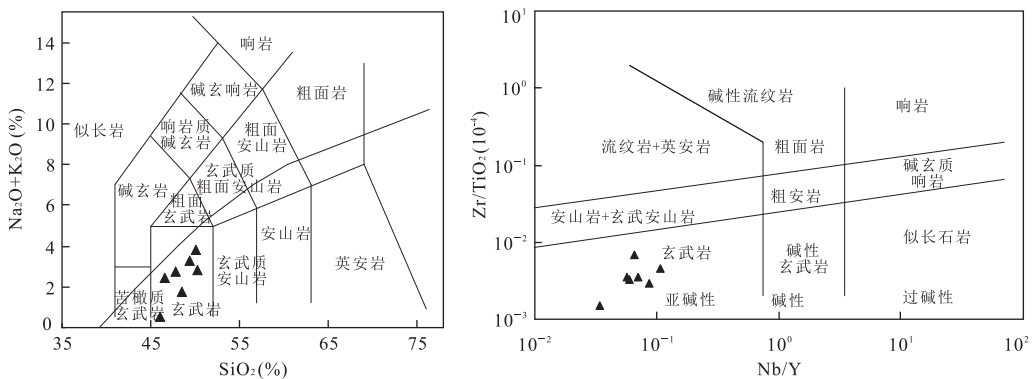
图 5 江错蛇绿岩 SiO 2 -Na 2 O+K 2 O 和 Nb/Y vs. Zr/TiO 2 岩石分类
