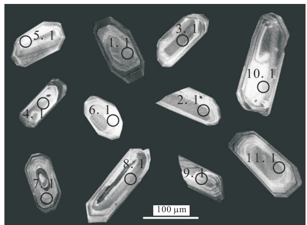
图 8 江错蛇绿岩中辉长岩锆石 CL 图像
