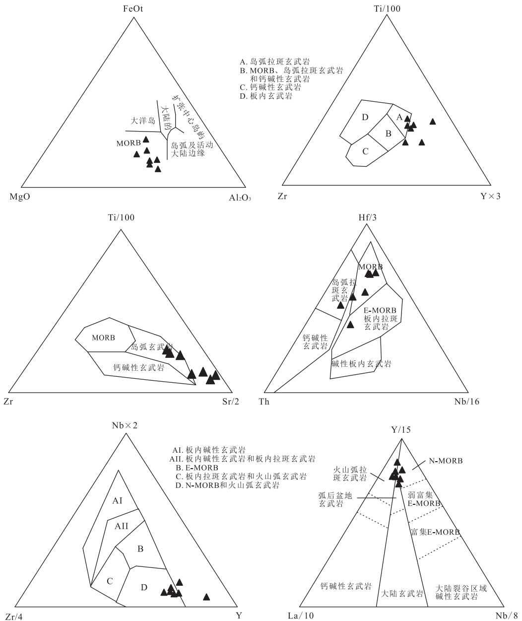
图 10 江错蛇绿岩微量元素构造环境判别图解
