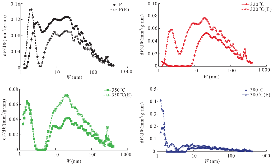
图 1 抽提前后样品的中、大孔孔径分布对比(低成熟至成熟阶段样品)
